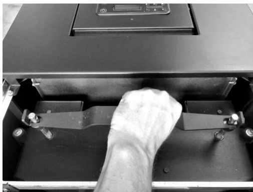
Fig. 26 - Palanca para la limpieza de los dispositivos de turbulencia
