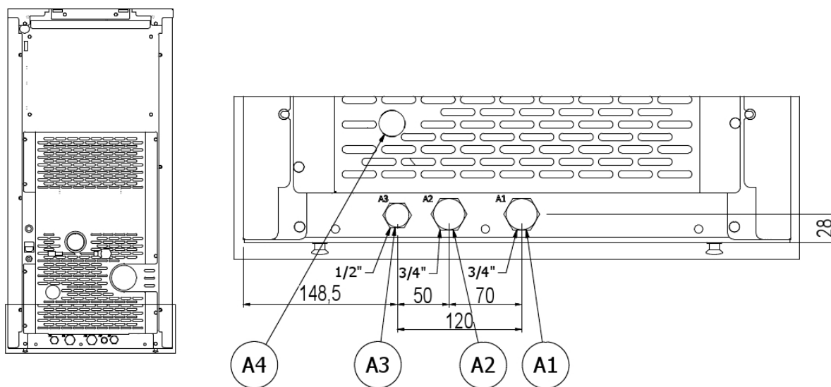
Fig. 34 - Aansluitschema (zonder SWW)
