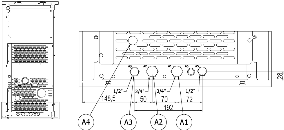
Fig. 35 - Aansluitschema met SWW
