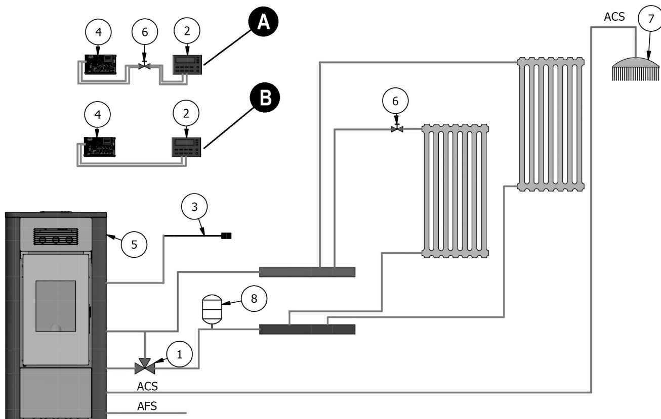
Fig. 40 - Configuratie 2
