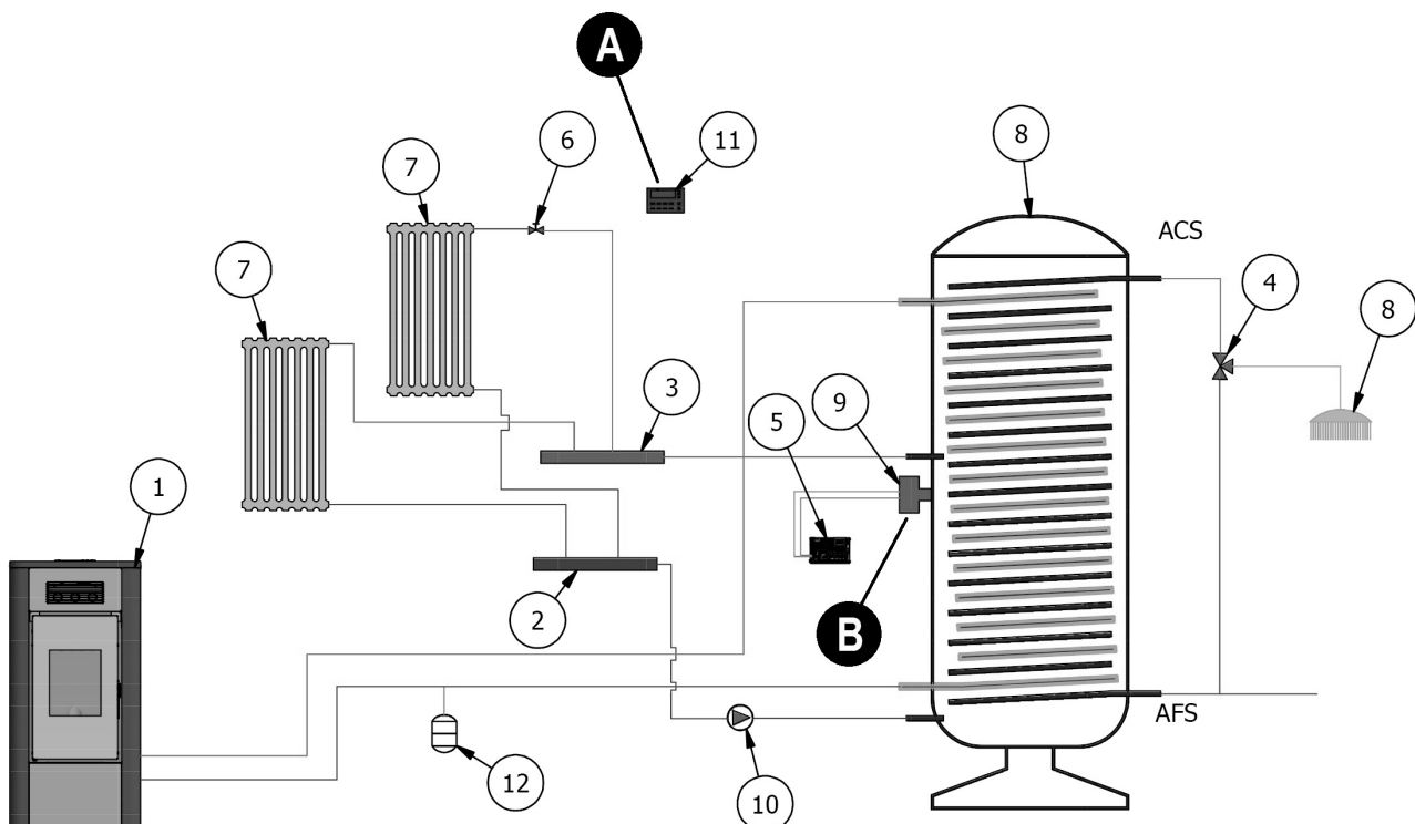
Fig. 43 - Configuratie 4
