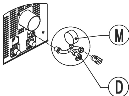
Fig. 37 - Terminal met vulkraan (D) en manometer (M)
