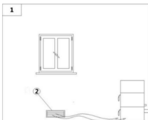
Fig. 10 - Directe luchttoevoer
