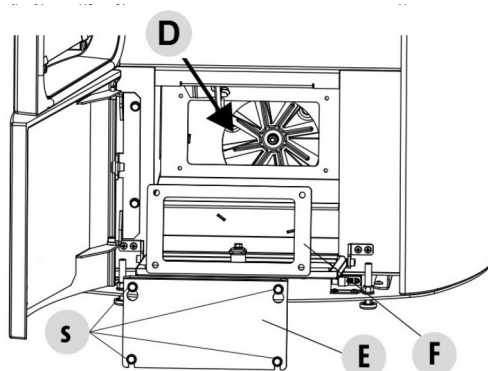
Fig. 54 - Reiniging onderste ruimte
