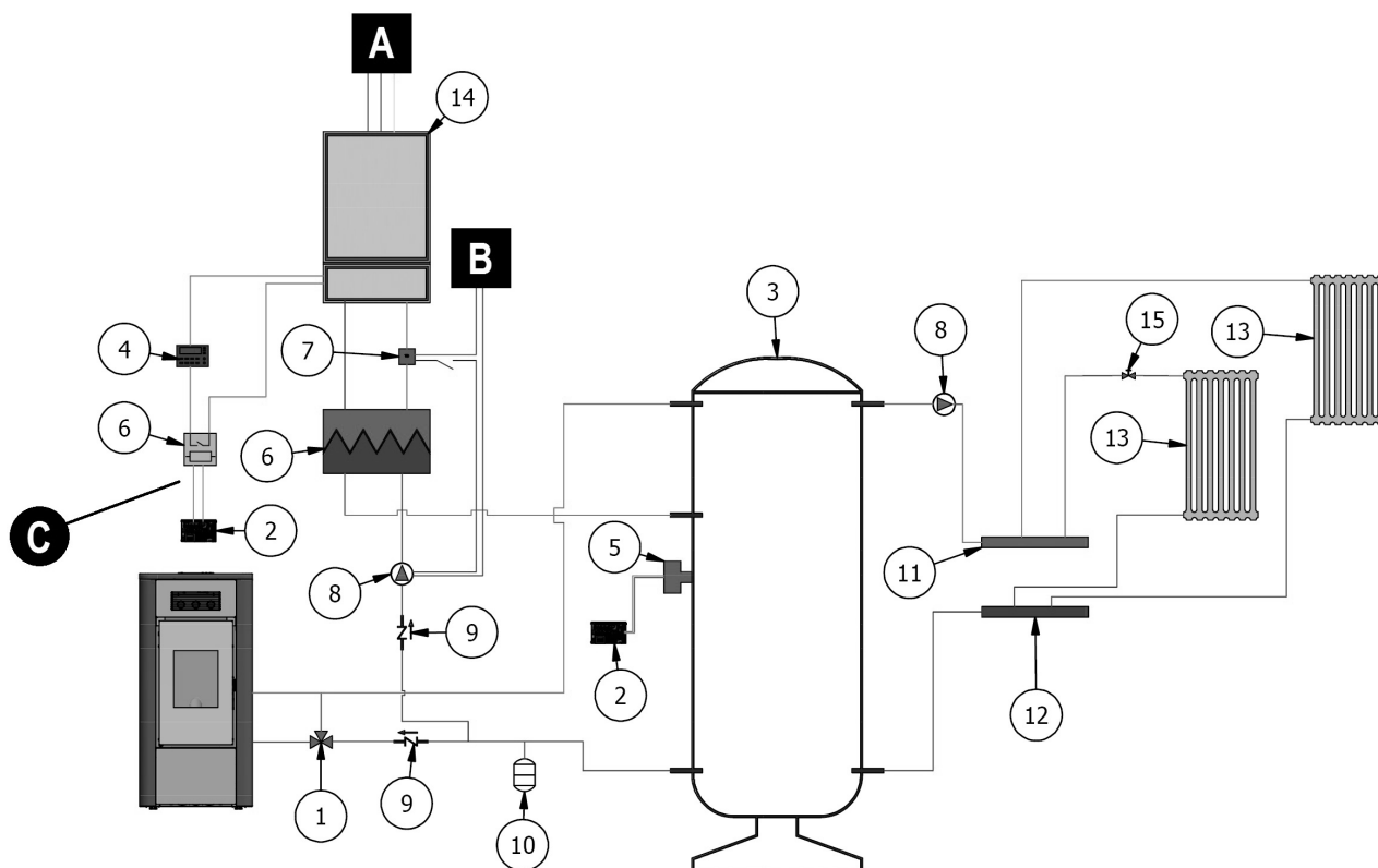
Fig. 45 - Configuratie met boiler en hulpketel aan muur
