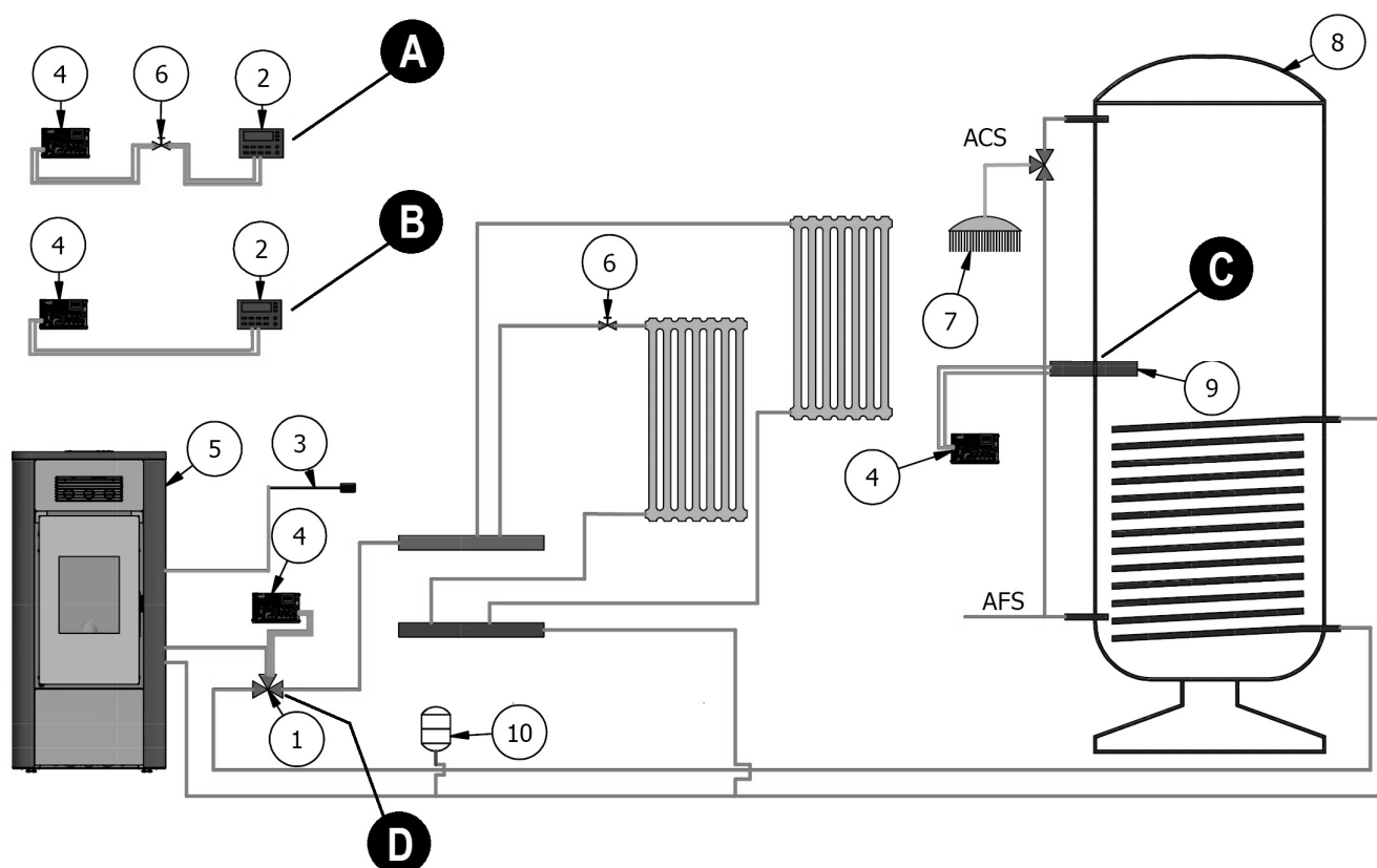
Fig. 42 - Configuratie 3
