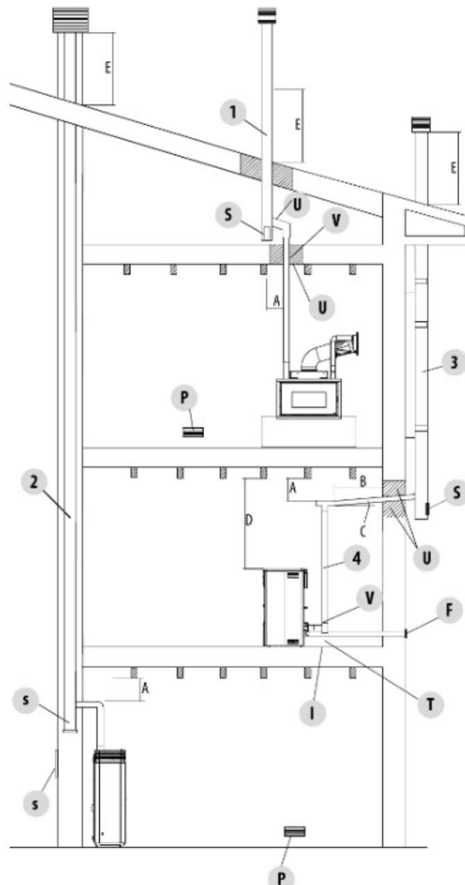
Fig. 13 - Rookkanaal
