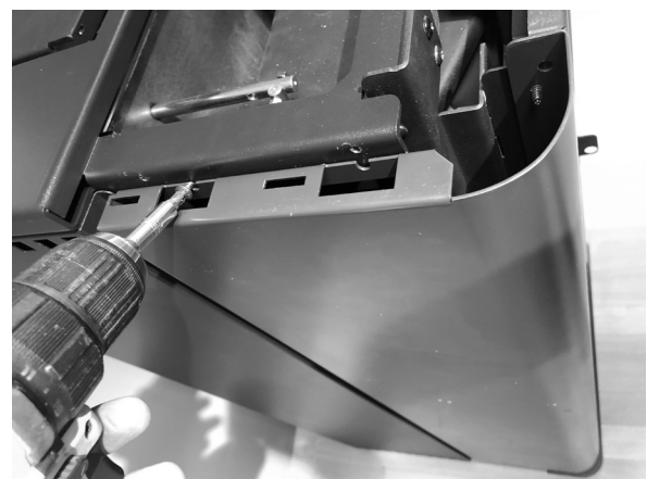
Fig. 22 - Zet de lijst vast
