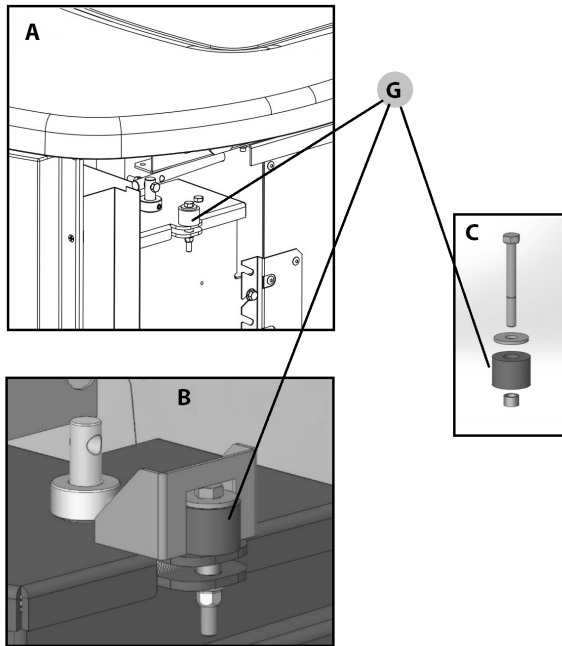
Fig. 65 - Rubbertje
