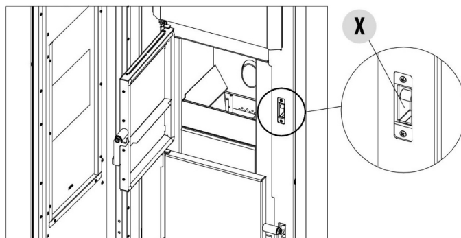
Fig. 55 - Sluiting deur
