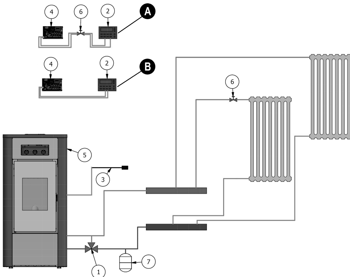
Fig. 39 - Configuratie 1
