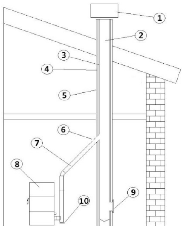
Fig. 5 - Onderdelen van de schoorsteen
