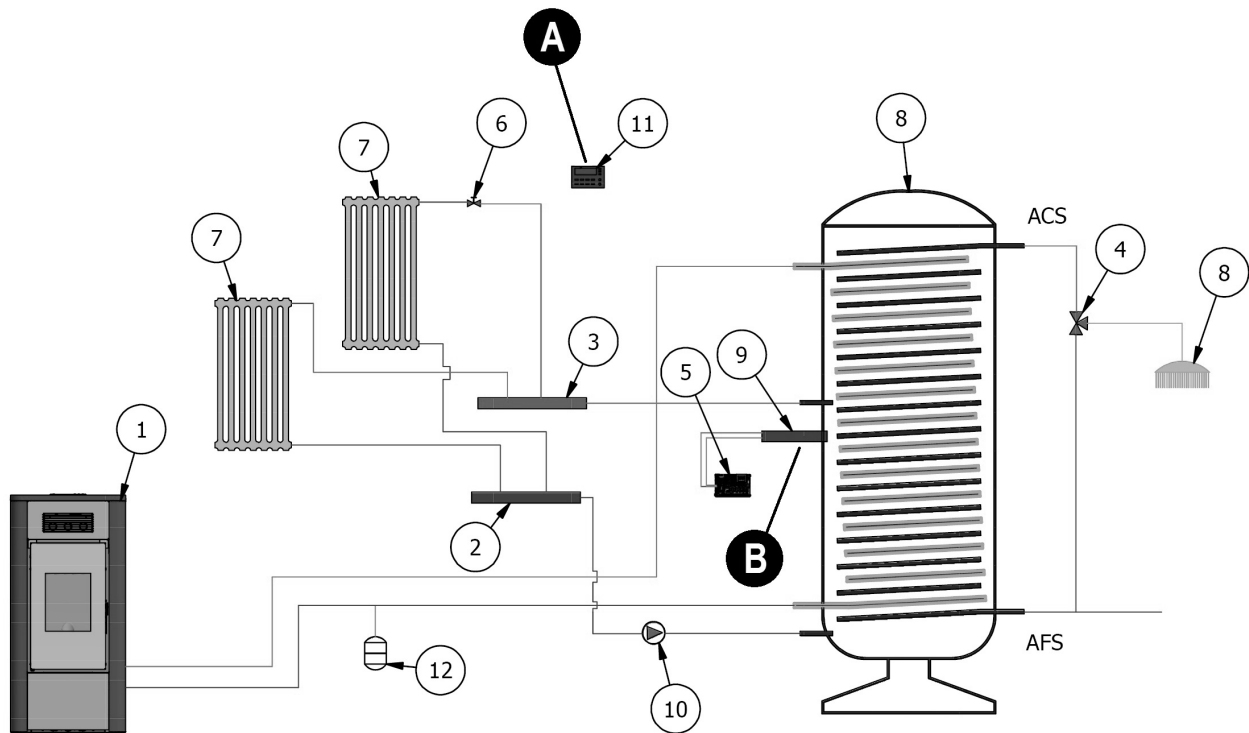
Fig. 44 - Configuratie 5
