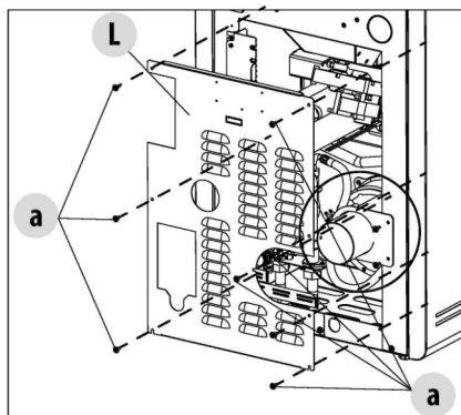
Fig. 50 - Achterpaneel
