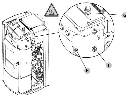
Fig. 38 - Manuele ontluchtingsklep (onder de top) Idro Prince 3 16-23-23 H2O, Aquos 3 16-23-23 H2O, Idron 16-22 Airtight, Hidrofire 22.8
