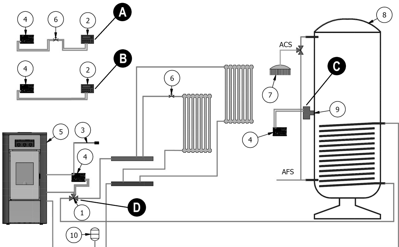
Fig. 41 - Configuratie 2
