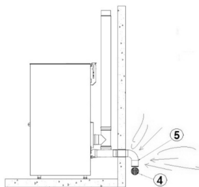
Fig. 11 - Luchtinlaat voor installatie met hermetisch gesloten kamer
