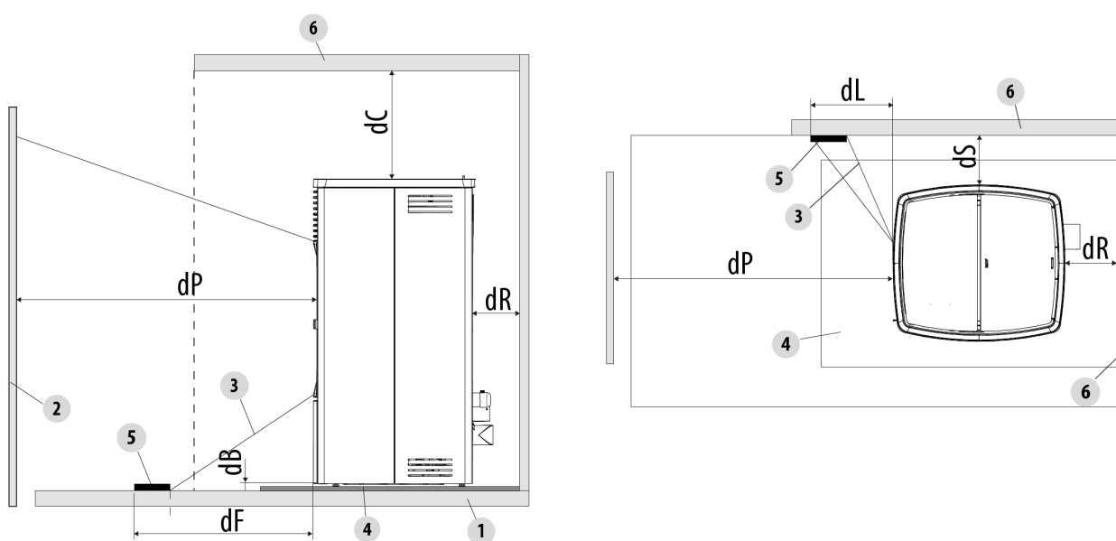
Fig. 14 - Veiligheidsafstand tot brandbaar materiaal (mm)
