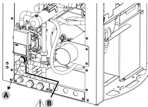
Fig. 37 - Soupape de décharge
