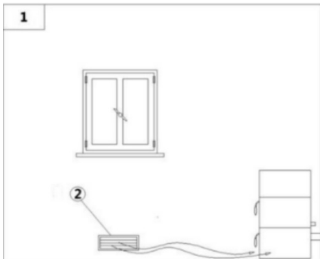
Fig. 11 - Entrée d'air directe
