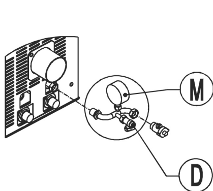
Fig. 38 - Terminal avec robinet de remplissage (D) et manomètre (M)
