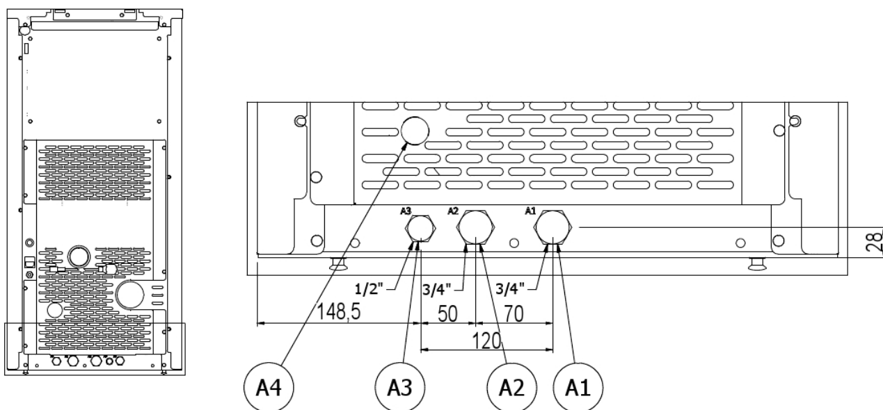
Fig. 35 - Schéma de raccordement (sans ECS)
