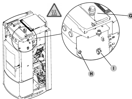
Fig. 39 - Purgeur manuel (situé sous le couvercle) (Idro Prince 3 16-23-23 H2O, Aqos 3 16-23-23 H2O, Idron 16-22 Airtight, Hidrofire 22.8)
