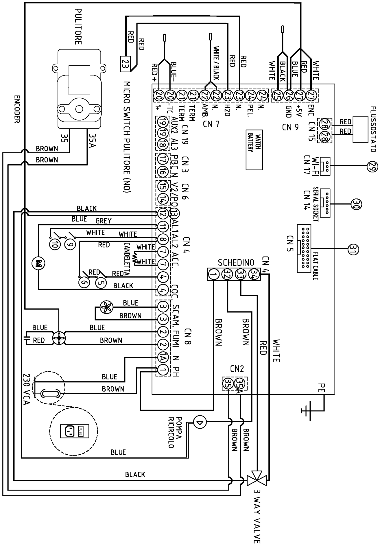
Fig. 69 - Scheda elettronica con kit sanitario
