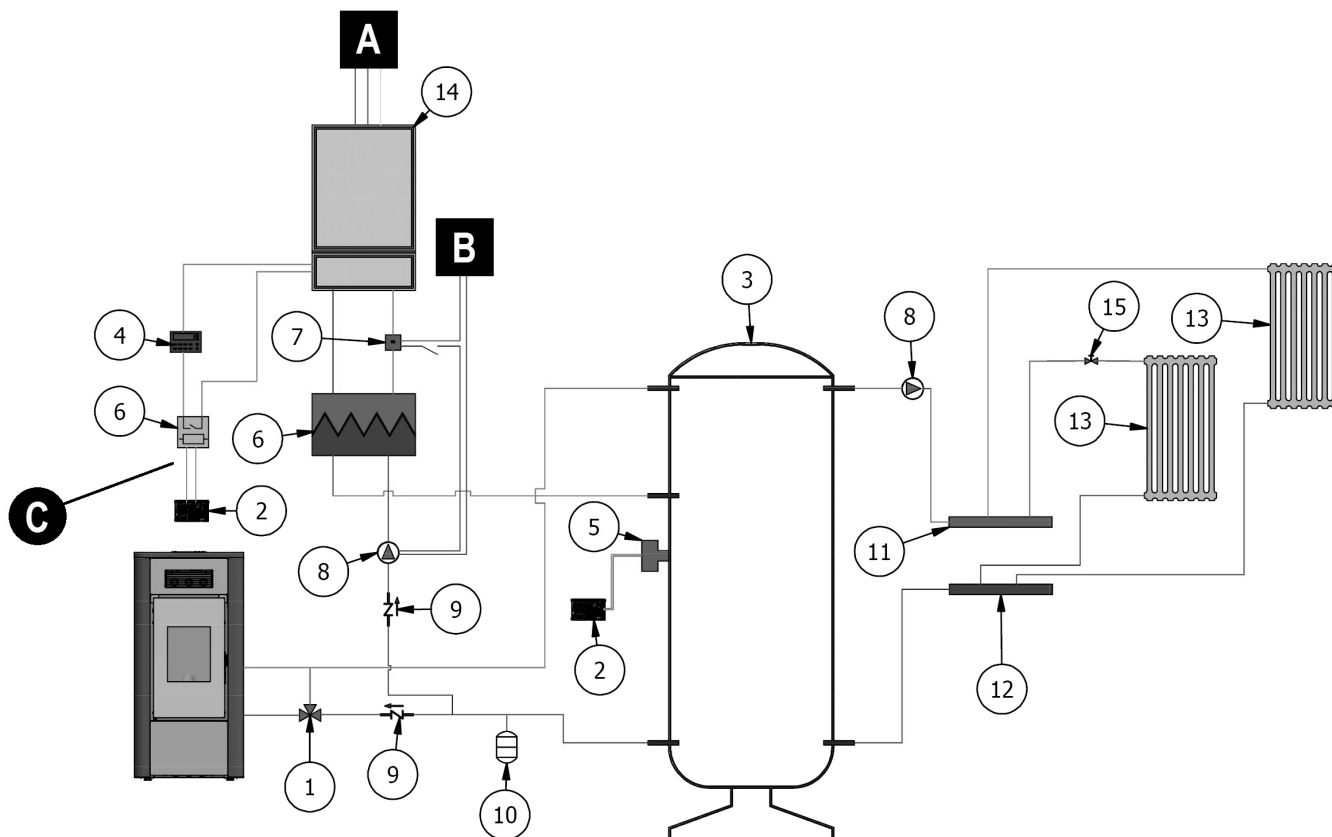
Fig. 46 - Configuration avec chauffe-eau et chaudière de secours murale
