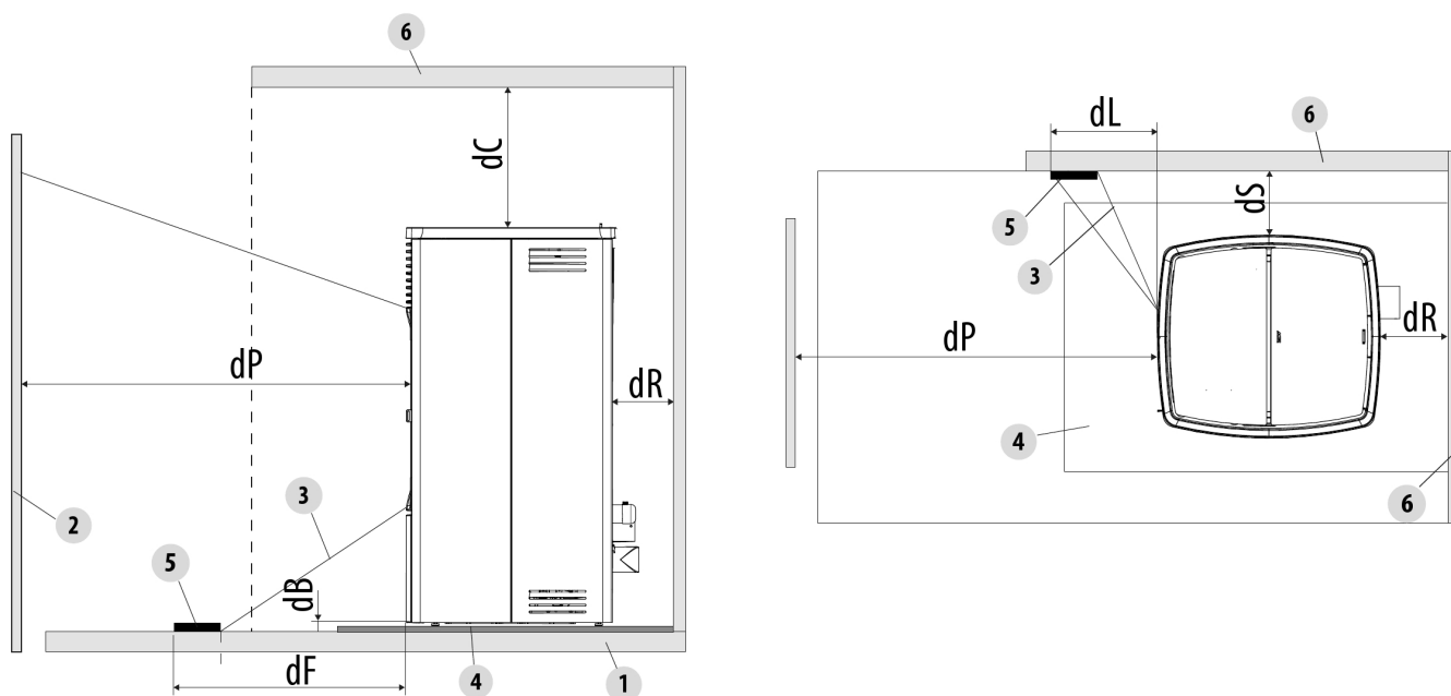
Fig. 15 - Distances de sécurité
