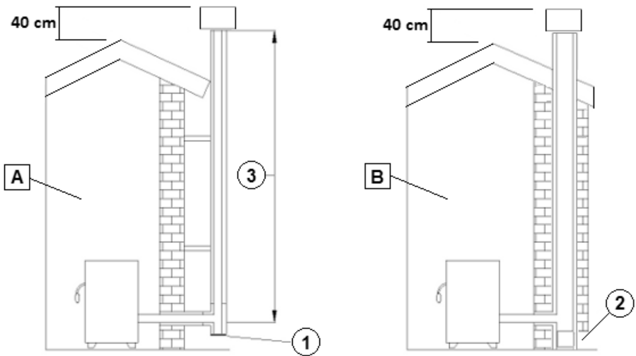
Fig. 6 - Conduit de fumées
