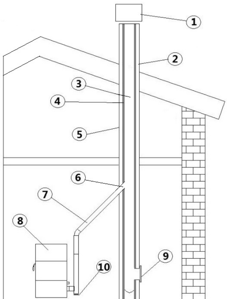
Fig. 5 - Composants de la cheminée
