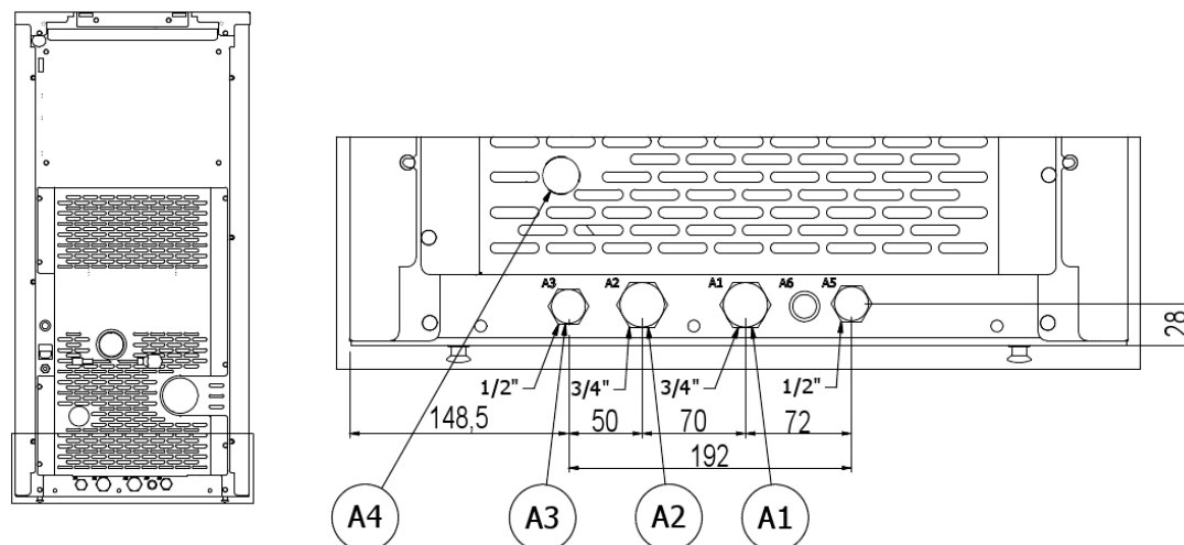
Fig. 36 - Schéma de raccordement avec ECS
