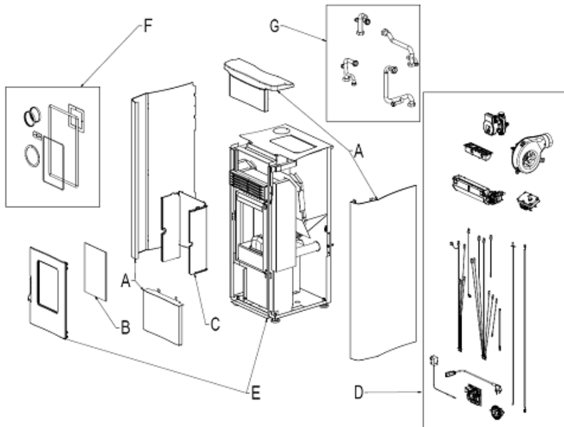
Fig. 1 - Esploso
