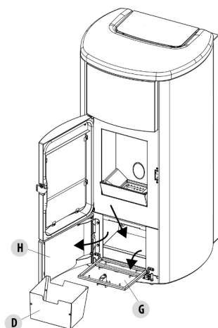
Fig. 24 - Rimozione cassetto
