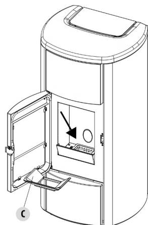
Fig. 25 - Rimozione braciere
