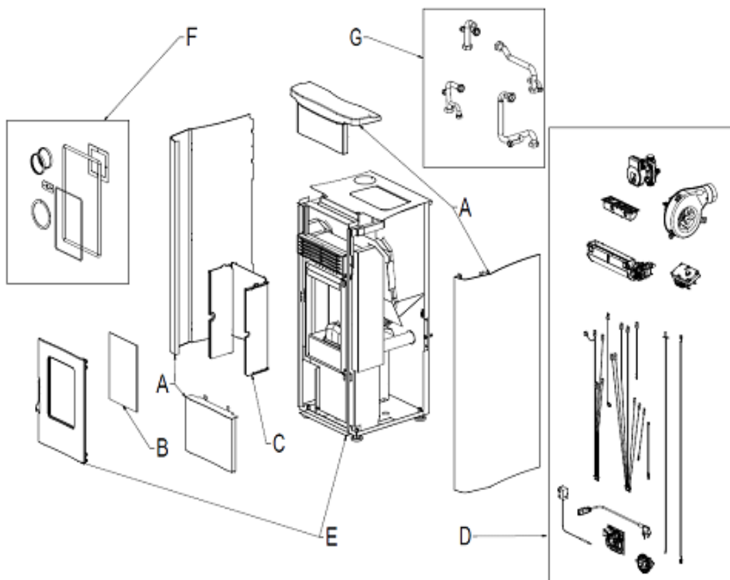
Fig. 1 - Geëxplodeerde tekening
