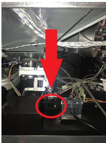
Fig. 43 - Manuele reset: achter het reservoir in de buurt van de stekker..
