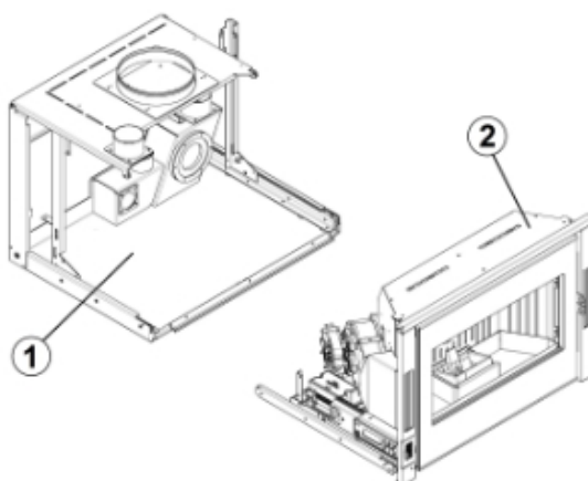
Fig. 25 - Structuur + machineromp
