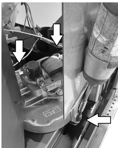
Fig. 100 - Pulizia 1
