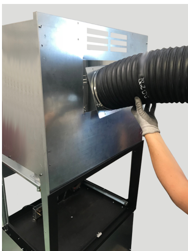
Fig. 67 - Posizionamento tubo flessibile
