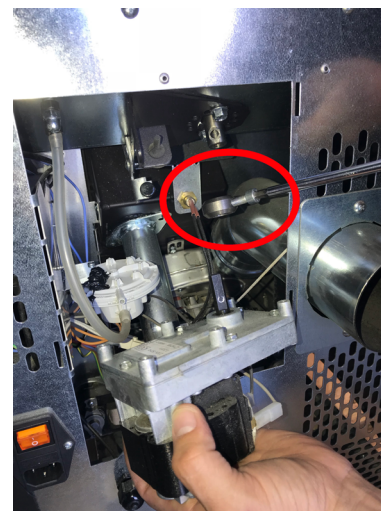
Fig. 93 - Rimozione motoriduttore
