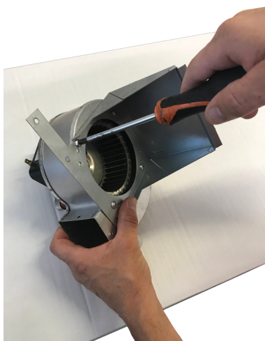
Fig. 42 - Rimuovere viti
