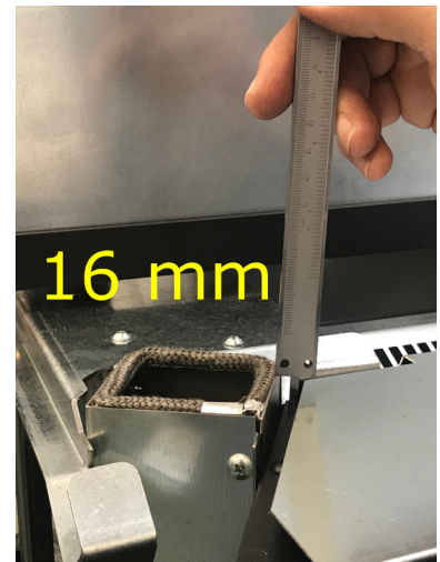
Fig. 46 - Sporgenza del deviatore aria
