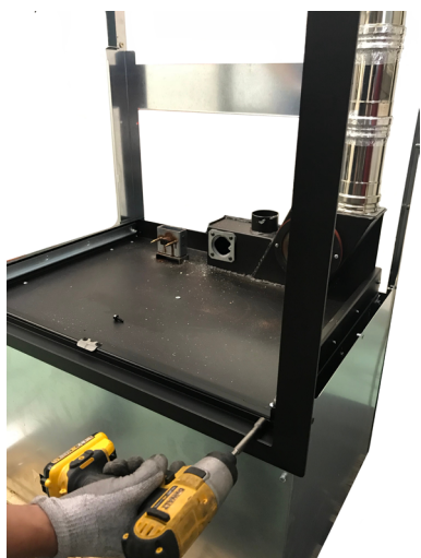
Fig. 76 - Fissaggio frontale
