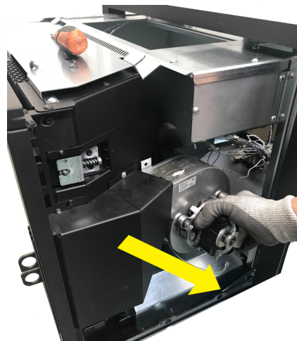
Fig. 99 - Rimuovere ventilatore
