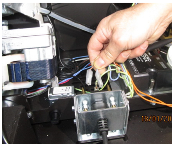
Fig. 88 - Disconnessione faston (blu - marrone)
