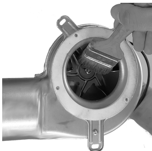
Fig. 101 - Pulizia 2
