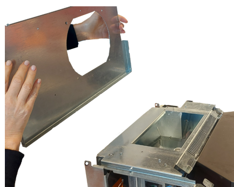
Fig. 52 - Rimuovi coperchio 2
