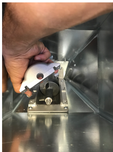
Fig. 92 - Rimozione guscio
