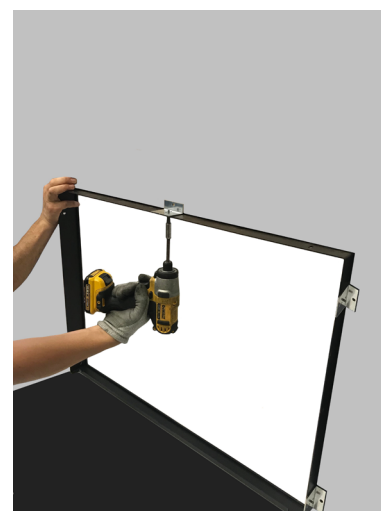
Fig. 78 - Fissaggio posteriore 2
