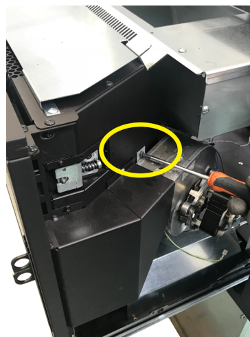
Fig. 97 - Rimuovere vite 1
