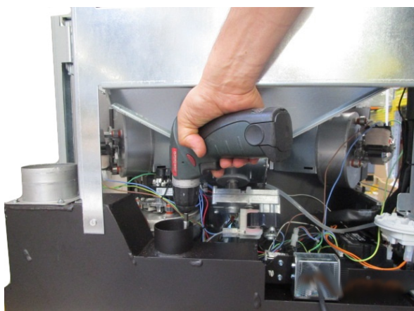
Fig. 32 - Rimozione anello 1
