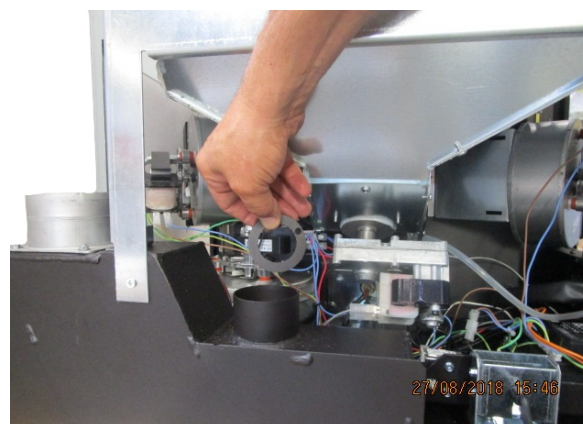
Fig. 33 - Rimozione anello 2
