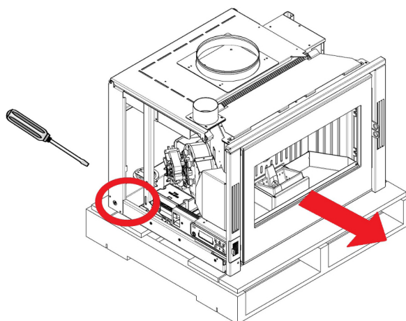
Fig. 1 - Rimozione viti
