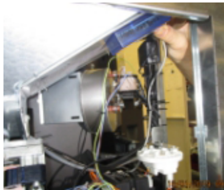
Fig. 90 - Fissaggio modulo Wi-Fi
