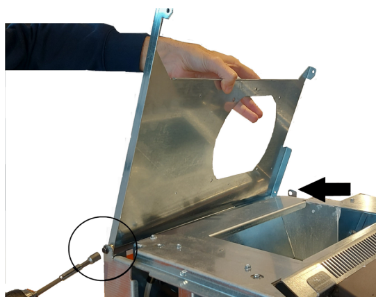
Fig. 51 - Rimuovi coperchio 1
