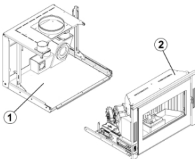
Fig. 25 - Struttura + corpo macchina
