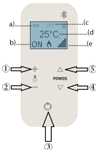
Fig. 41 - Telecomando con termostato
