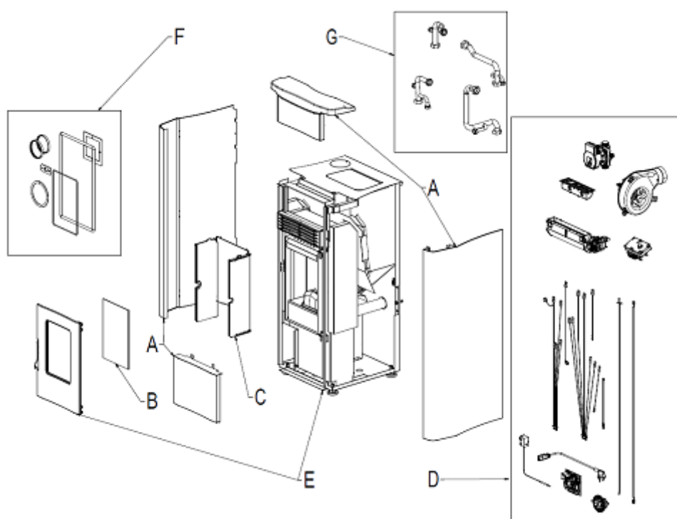
Fig. 1 - Esploso
