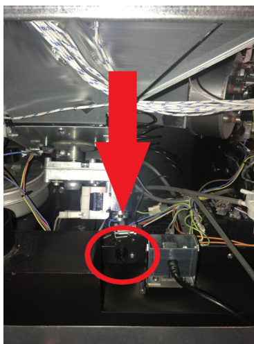
Fig. 43 - Riarmo manuale: si trova dietro al serbatoio, vicino alla spina di alimentazione
