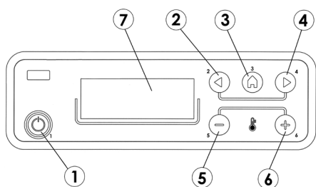
Fig. 8 - Bedieningspaneel
