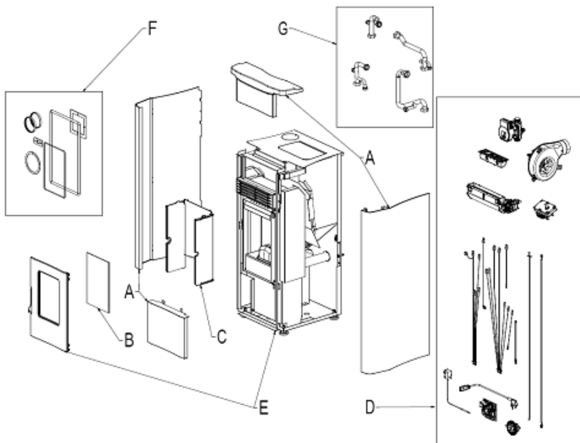
Fig. 1 - Esploso
