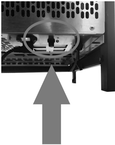
Fig. 30 - Riarmo manuale: si trova sotto la stufa FRAME
