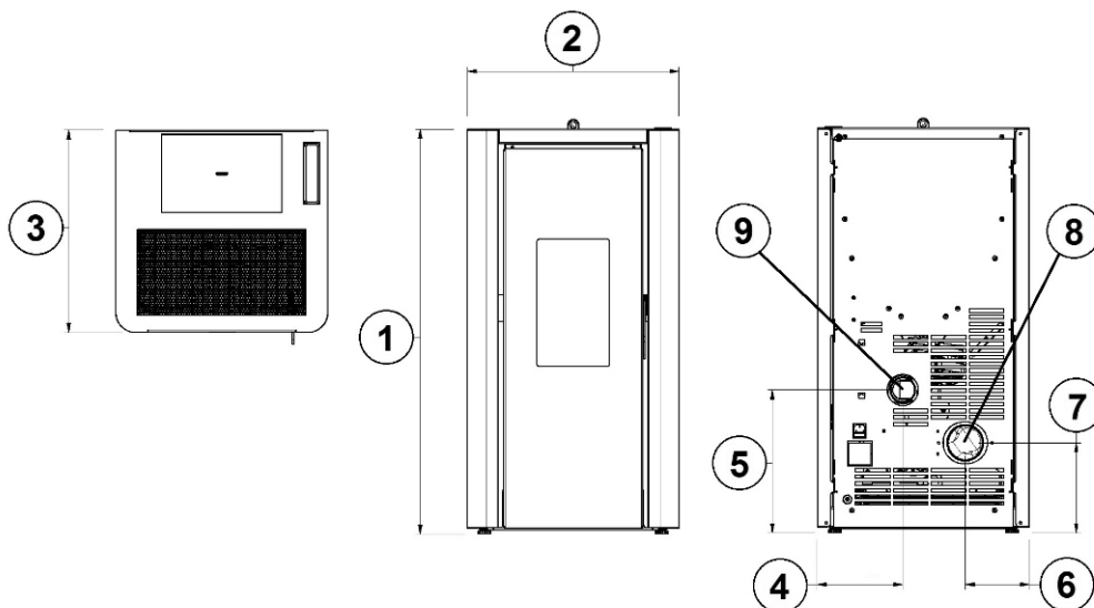
Fig. 14 - Dimensiones generales: INDIGO EVO
