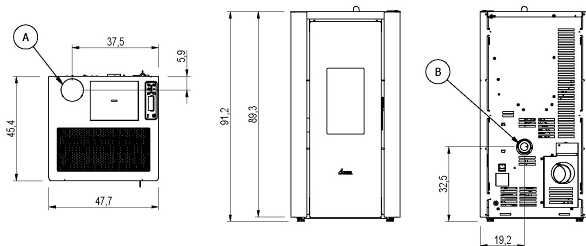
Fig. 16 - Dimensiones generales: CRISTAL3 7.0 UP
