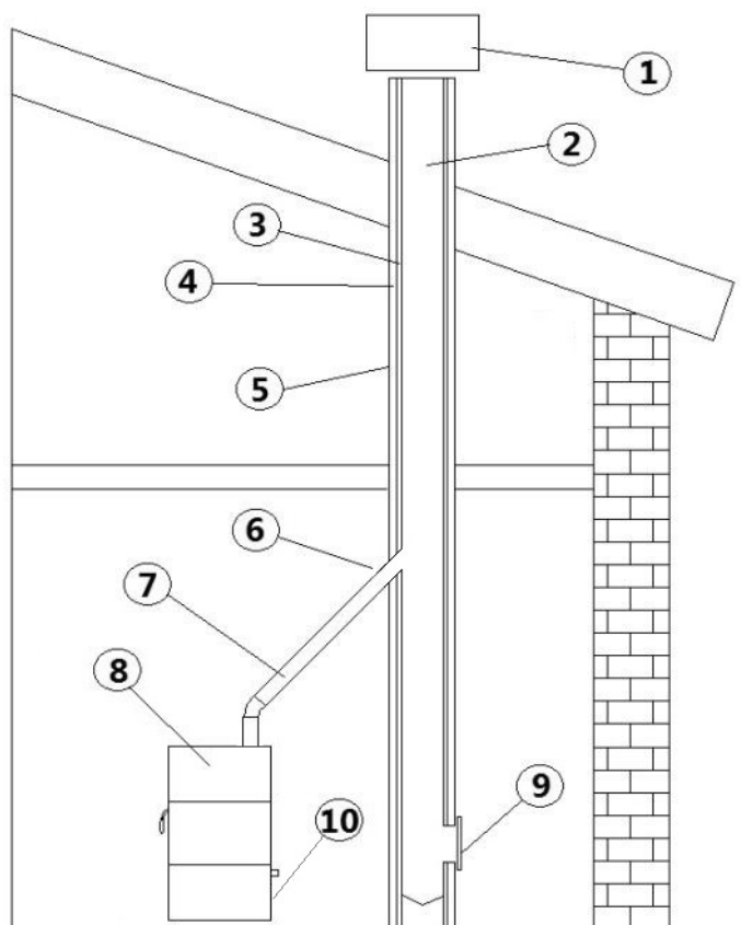
Fig. 2 - Componentes chimenea
