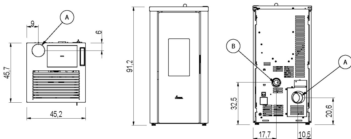
Fig. 15 - Dimensiones generales: VERA 7.0 UP
