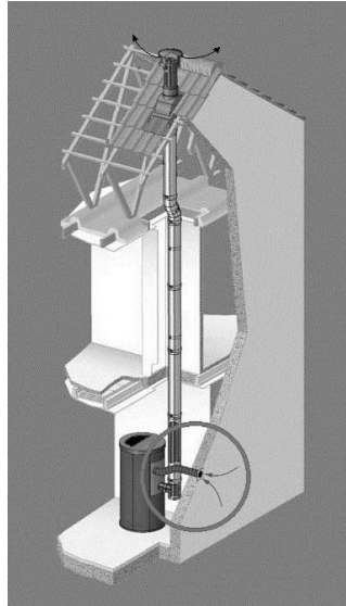
Fig. 11 - Installation en chambre étanche
