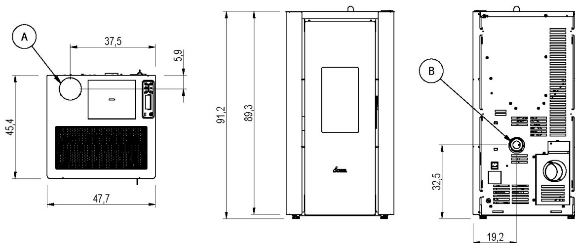
Fig. 17 - Dimensions générales: CRISTAL7.0 UP
