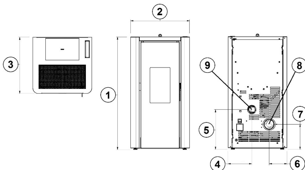
Fig. 15 - Dimensions générales: INDIGO EVO
