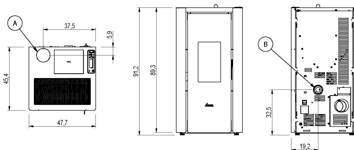
Fig. 14 - Dimensioni generali: CRISTAL 7.0 UP
