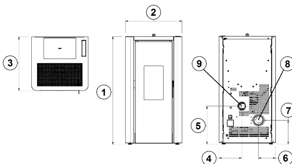
Fig. 12 - Dimensioni generali: INDIGO EVO
