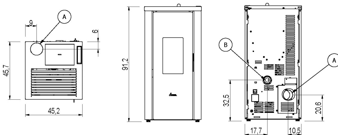
Fig. 13 - Dimensioni generali: VERA 7.0 UP
