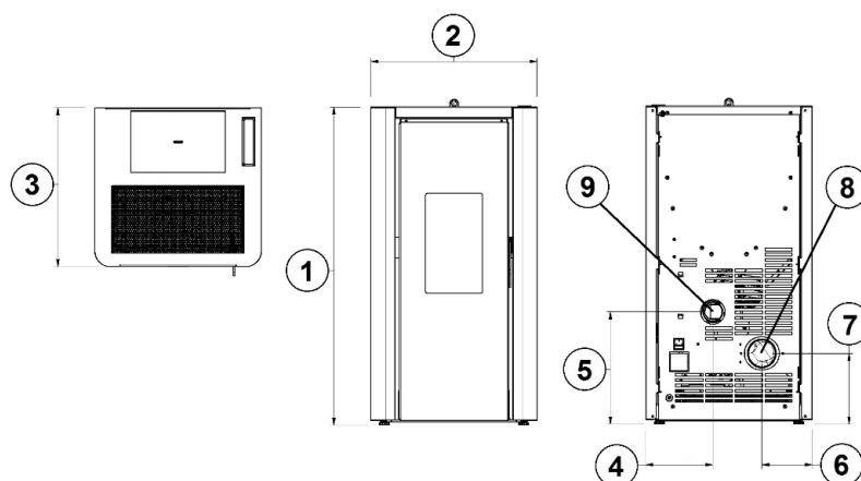
Fig. 35 - Dimensions générales: INDIGO EVO 7
