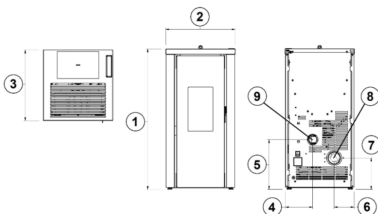
Fig. 21 - Dimensions générales: LORD 7 - 7.0
