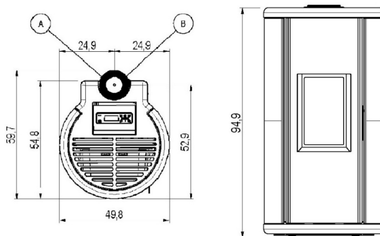
Fig. 26 - Dimensions générales: SOUND3 SUP - 7UP
