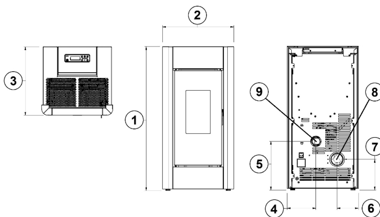
Fig. 22 - Dimensions générales: SWEET³ 7 - 7.0
