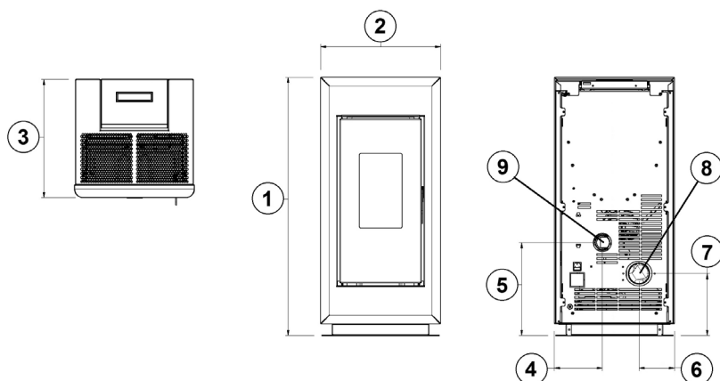
Fig. 31 - Dimensions générales: ACCENT AIRTIGHT
