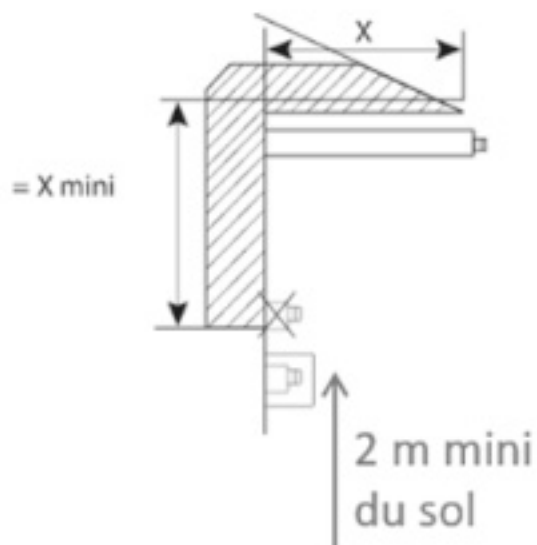
Fig. 14 - Rebord de toit
