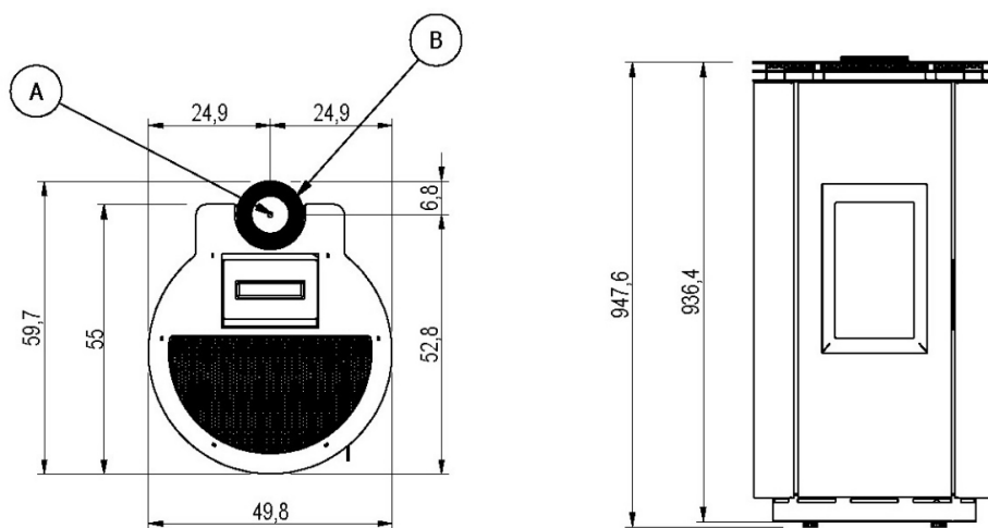
Fig. 29 - Dimensions générales: FLOYD 5.0 - 7.0
