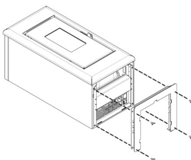
Fig. 56 - Montage du socle
