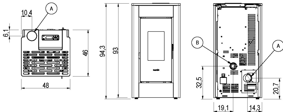
Fig. 25 - Dimensions générales: SHARP AIRTIGHT - LEE AIRTIGHT
