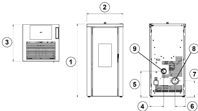
Fig. 32 - Dimensions générales: VERA 7 - 7.0
