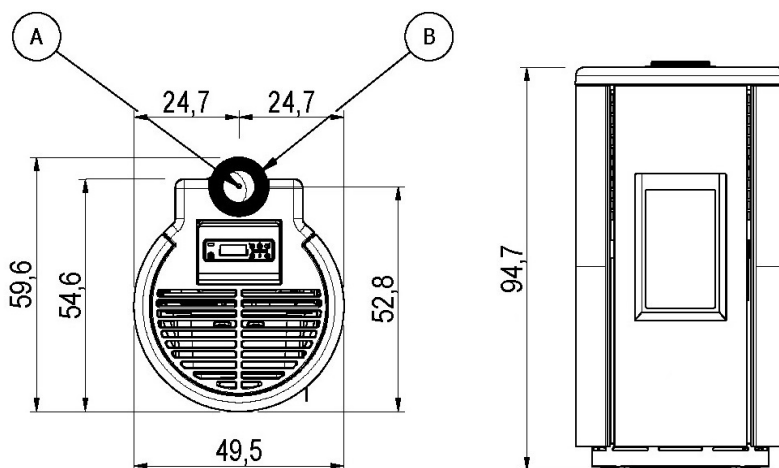
Fig. 28 - Dimensions générales: CHROME 5-7 AIRTIGHT - ROUND 5-7 AIRTIGHT
