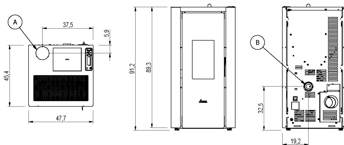
Fig. 34 - Dimensions générales: CRISTAL7.0 UP
