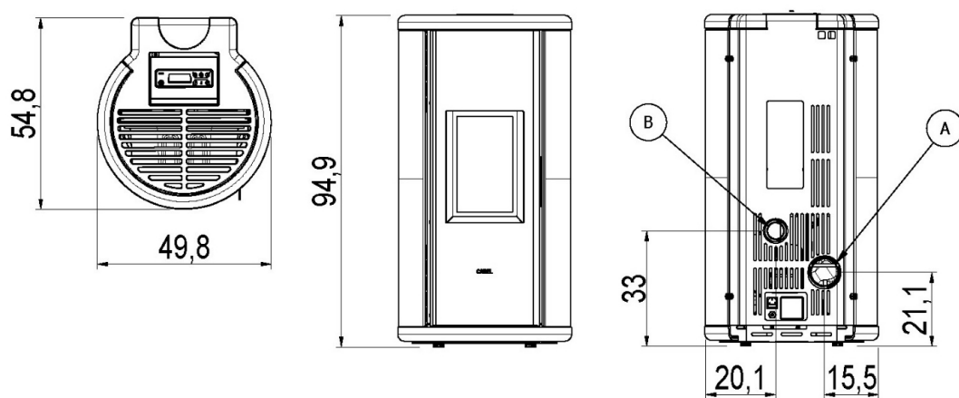
Fig. 27 - Dimensioni generali: SOUND 5PS - 7PS
