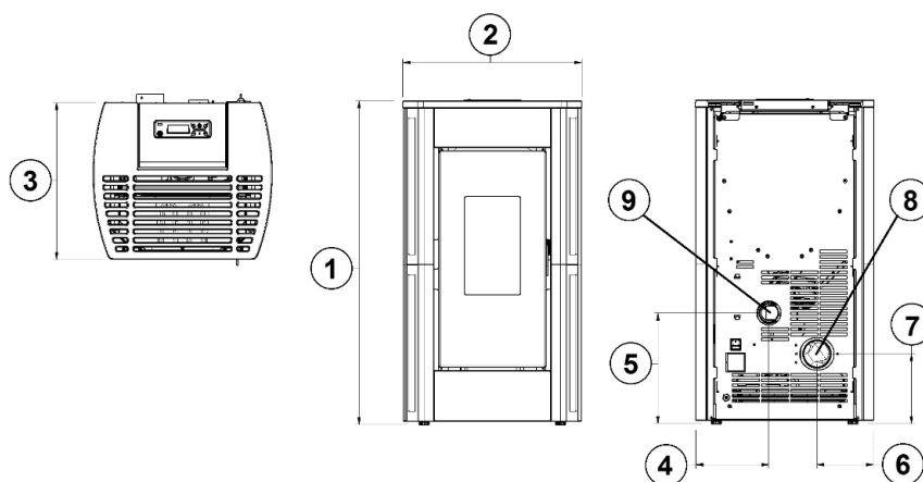
Fig. 23 - Dimensions générales: PERLA³ 7 - 7.0
