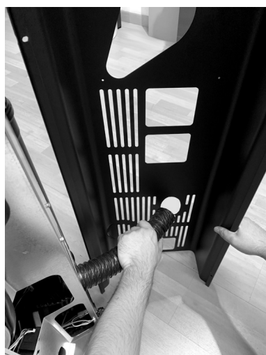
Fig. 68 - Passage du tuyau flexible 2
