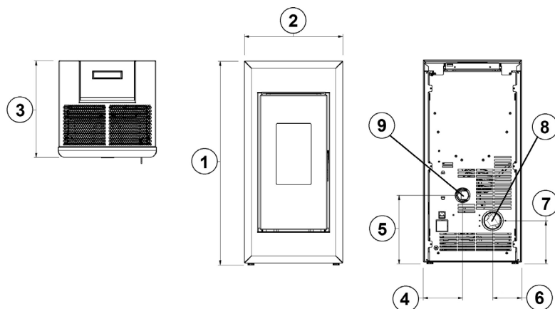
Fig. 30 - Dimensions générales: ONE/BEAM AIRTIGHT
