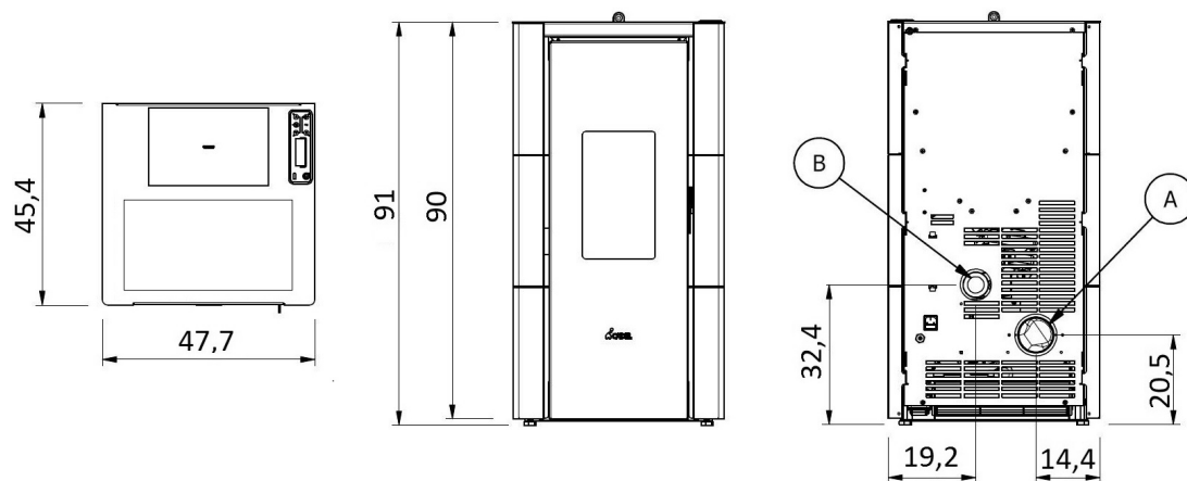
Fig. 24 - Dimensions générales: CRISTAL³ 7 - 7.0
