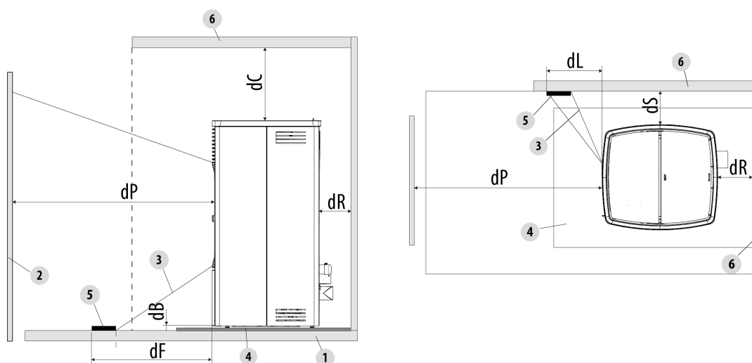
Fig. 20 - Distances de sécurité
