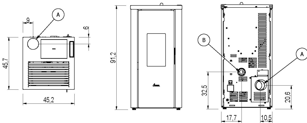
Fig. 33 - Dimensions générales: VERA 7.0 UP
