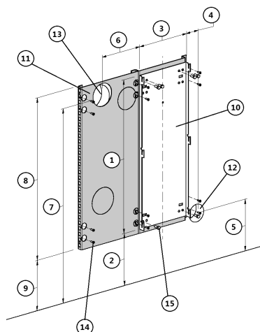
Fig. 20 - Fijación en pared inflamable
