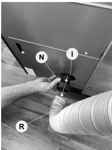
Fig. 13 - Tubo flexible
