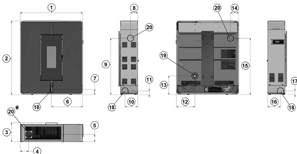
Fig. 25 - Dimensiones generales: Tile³ Plus
