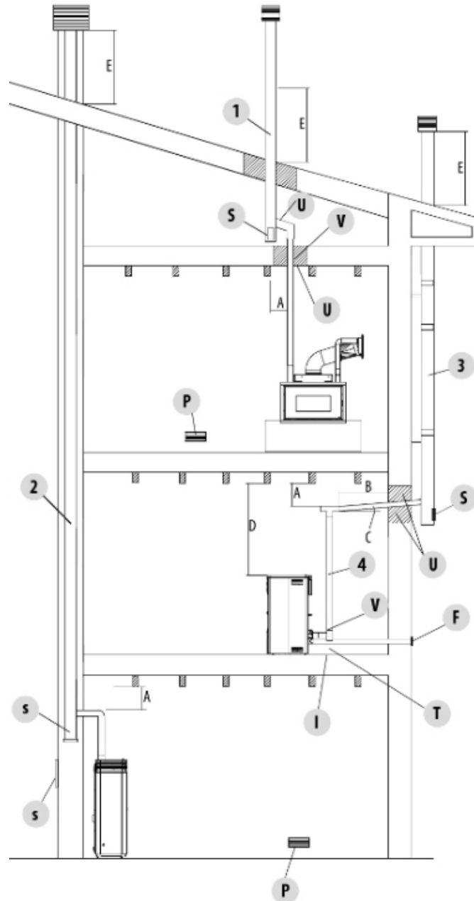
Fig. 16 - Sistema de evacuación de humos
