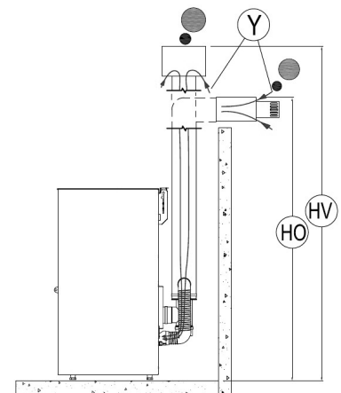
Fig. 15 - Conexiones del conducto de humos
