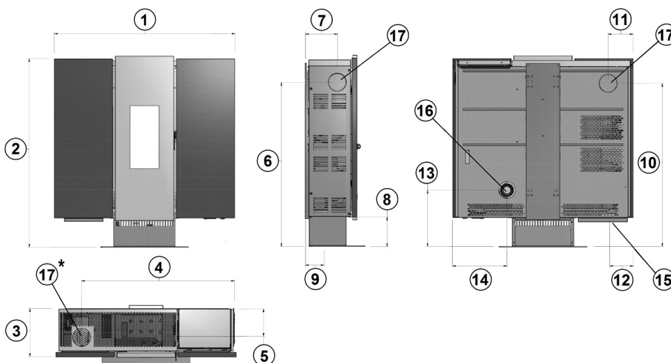
Fig. 22 - Dimensiones generales: Wall³ Plus
