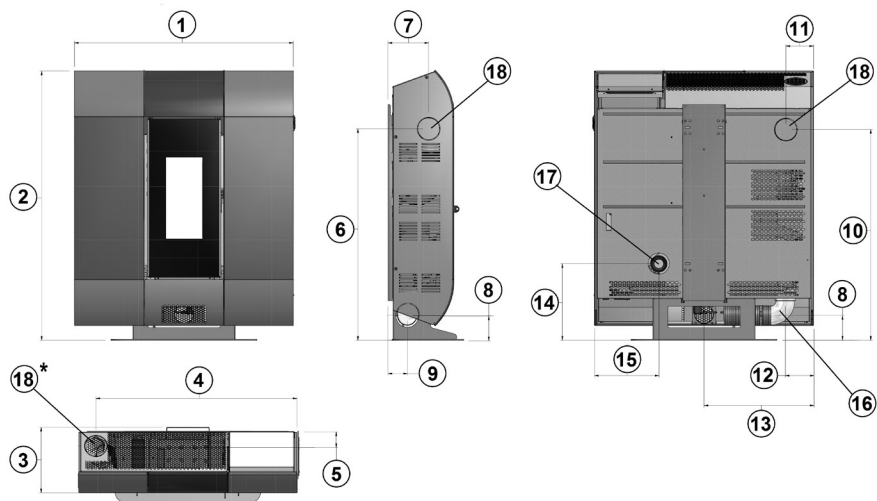
Fig. 23 - Dimensiones generales: Lean³ Plus
