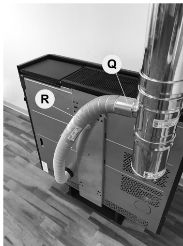
Fig. 14 - Conexiones
