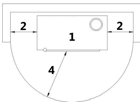
Fig. 18 - Instalación en pared
