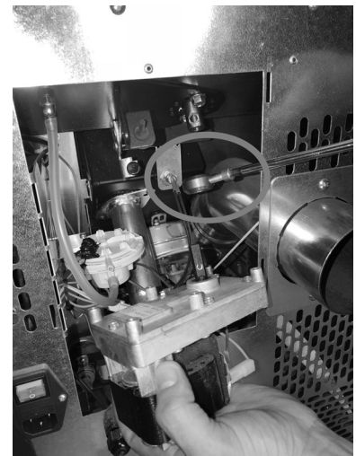
Fig. 52 - Extracción del motorreductor
