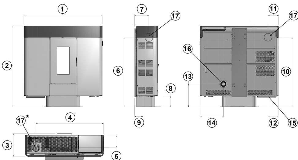
Fig. 24 - Dimensiones generales: Moon
