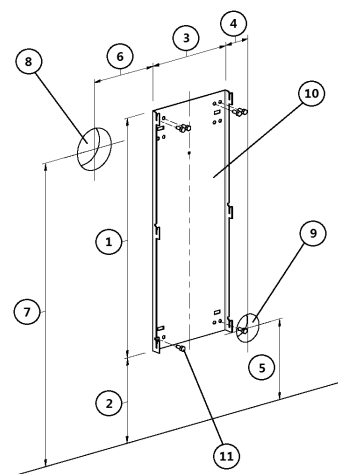
Fig. 19 - Fijación en pared no inflamable
