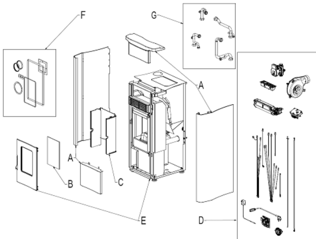
Fig. 1 - Geëxplodeerde tekening
