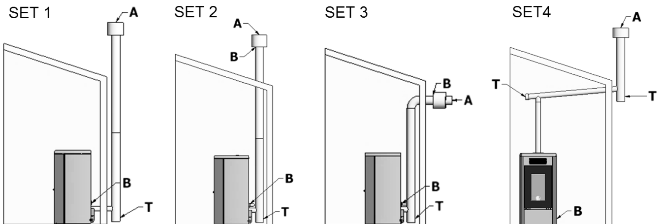
Fig. 25 - Voorbeelden Set
