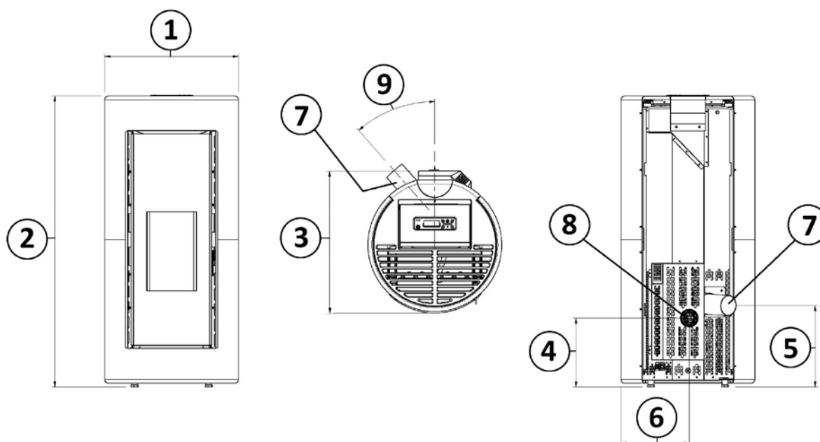
Fig. 16 - Dimensioni generali: Shell ® Ps
