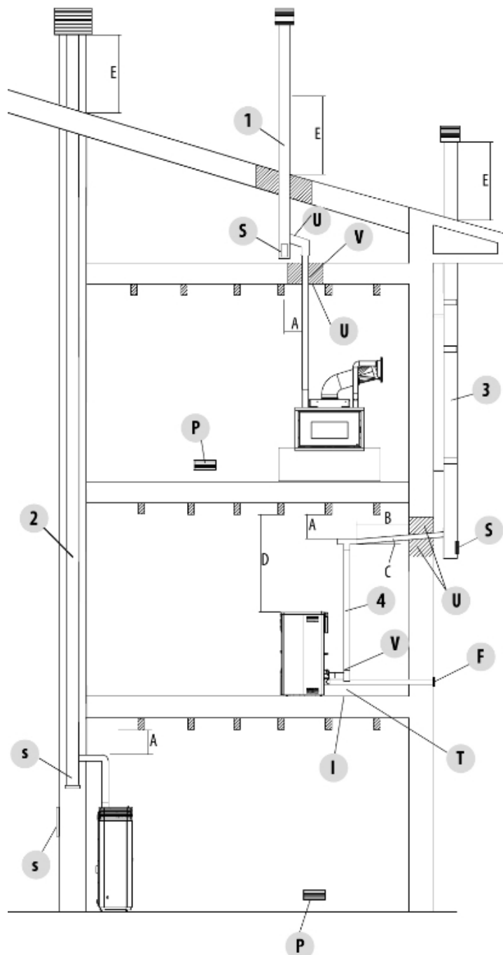
Fig. 14 - Canna fumaria
