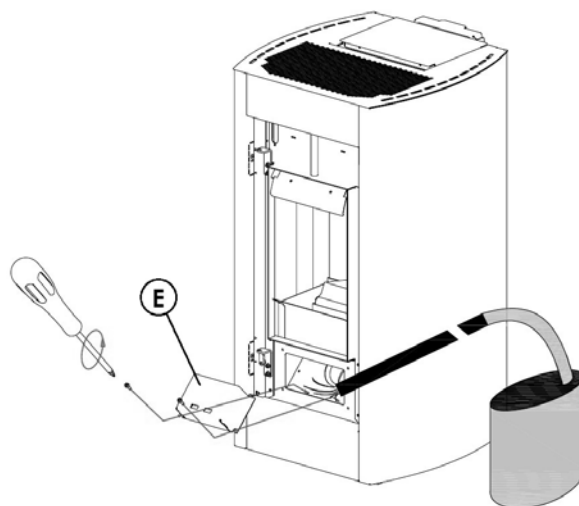
Fig. 41 - Pulizia
