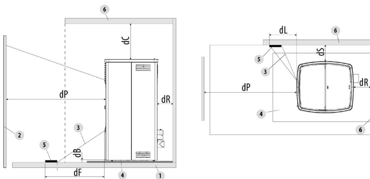
Fig. 15 - Distanze di sicurezza da materiale combustibile
