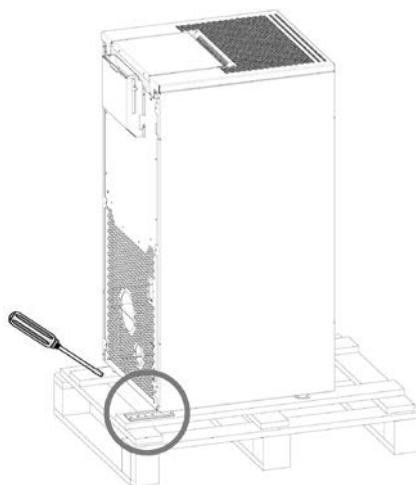
Fig. 1 - Rimozione staffe
