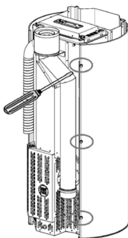
Fig. 28 - Togliere viti
