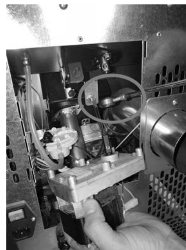
Fig. 46 - Rimozione motoriduttore
