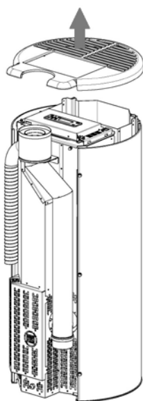
Fig. 27 - Rimozione top
