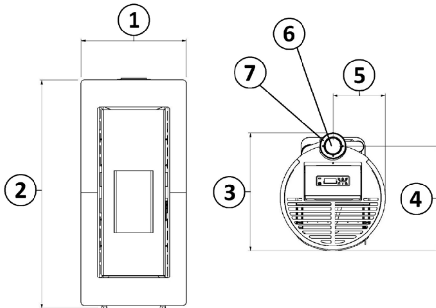
Fig. 17 - Dimensioni generali: Shelf Up
