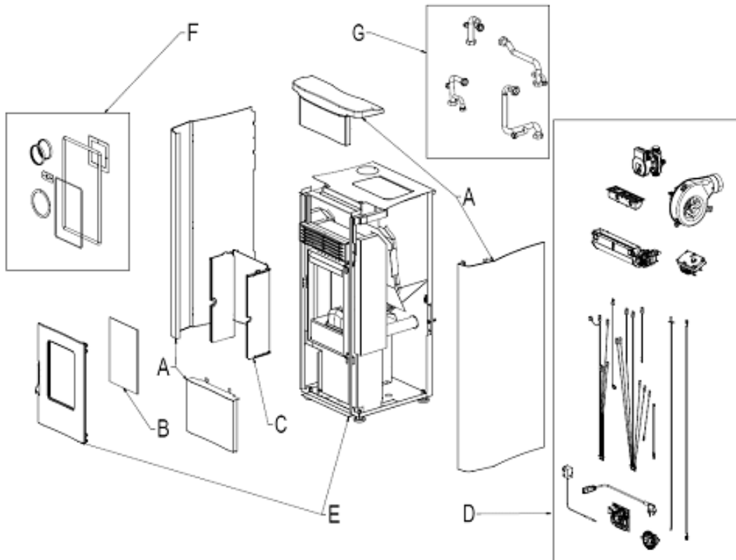
Fig. 1 - Geëxplodeerde tekening
