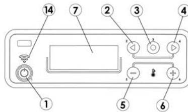
Fig. 8 - Bedieningspaneel (wi-fi)
