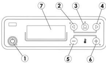
Fig. 7 - Bedieningspaneel
