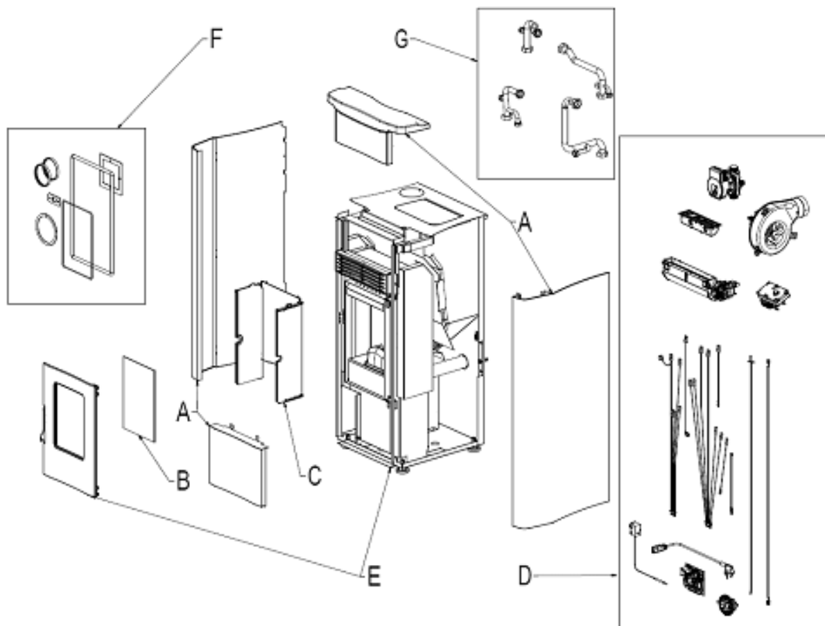
Fig. 1 - Dibujo explotado
