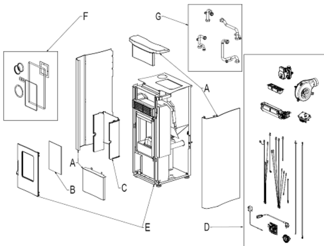
Fig. 1 - Dessin éclaté
