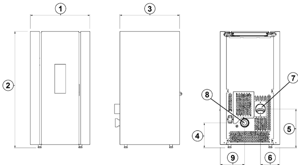
Fig. 26 - Algemene afmetingen: Titania Airtight - Venere Airtight
