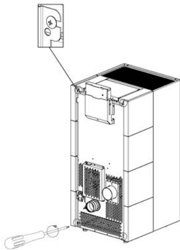
Fig. 62 - Draai de schroeven los
