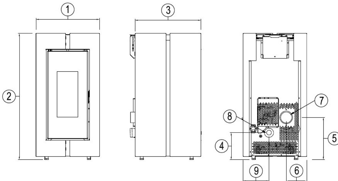
Fig. 17 - Algemene afmetingen: Tecna 3
