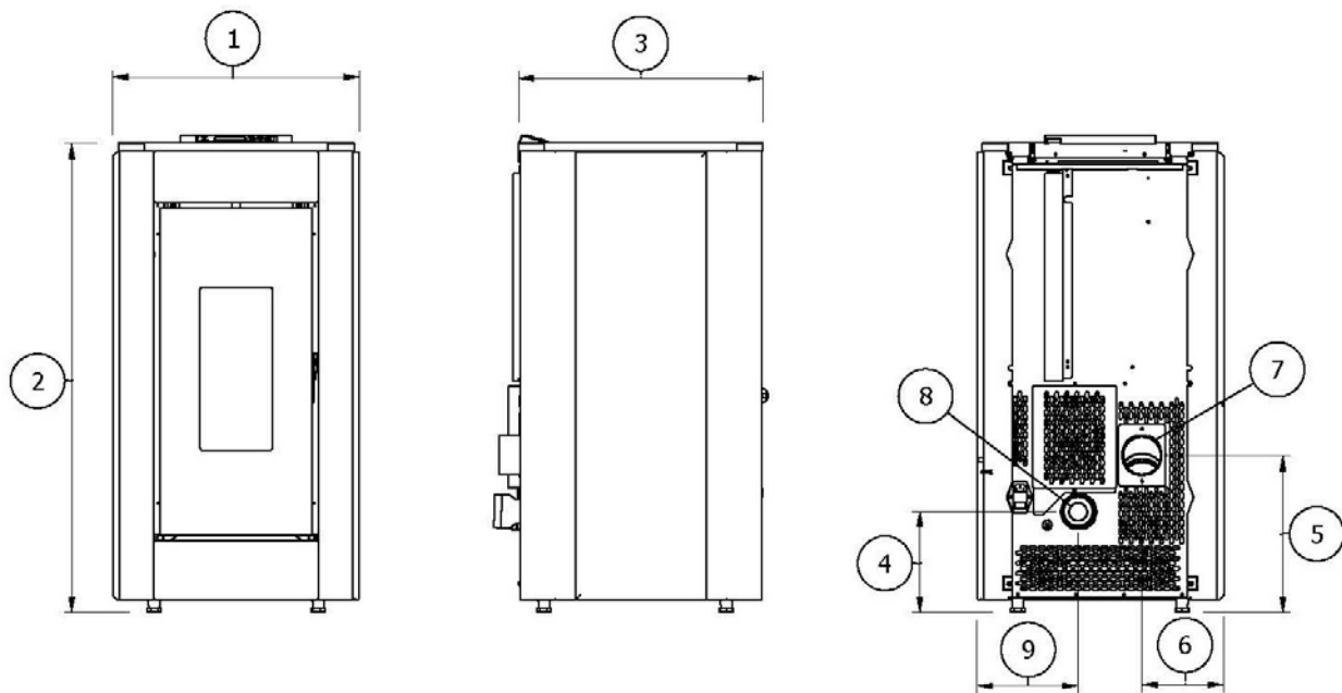
Fig. 25 - Algemene afmetingen: Pretty Airtight
