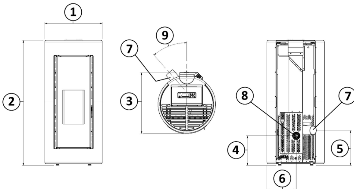
Fig. 27 - Algemene afmetingen: Shell P Ps
