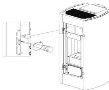
Fig. 57 - Verwijder de schroeven
