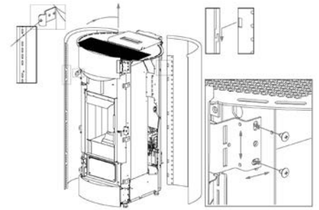
Fig. 61 - Regelingen
