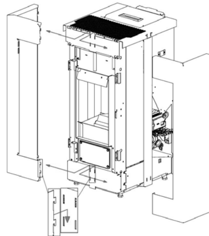
Fig. 55 - De zijpanelen losmaken
