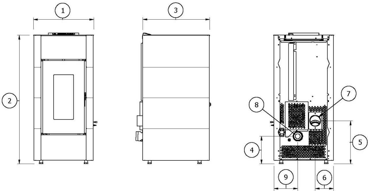
Fig. 24 - Algemene afmetingen: CristalP
