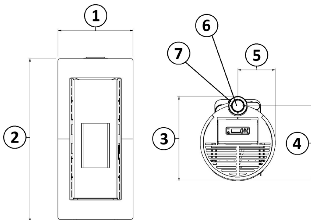
Fig. 28 - Algemene afmetingen: Shell P Up
