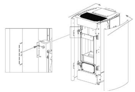
Fig. 58 - Verwijdering zijpanelen
