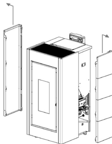
Fig. 63 - Verwijdering zijpanelen
