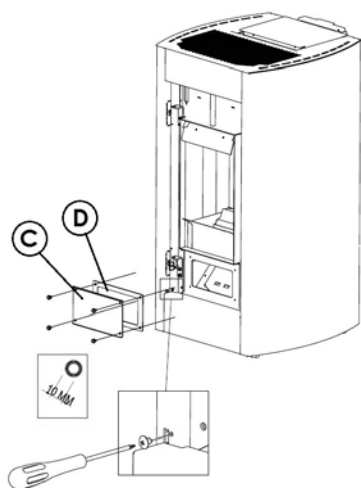
Fig. 88 - Verwijdering van de plaat
