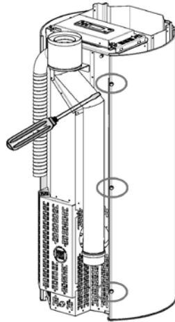
Fig. 73 - Schroeven verwijderen
