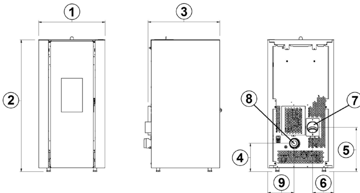
Fig. 30 - Algemene afmetingen: ELANE
