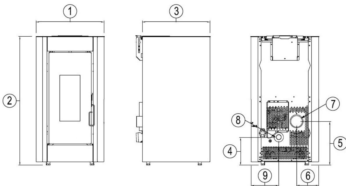
Fig. 19 - Algemene afmetingen: Kriss 3
