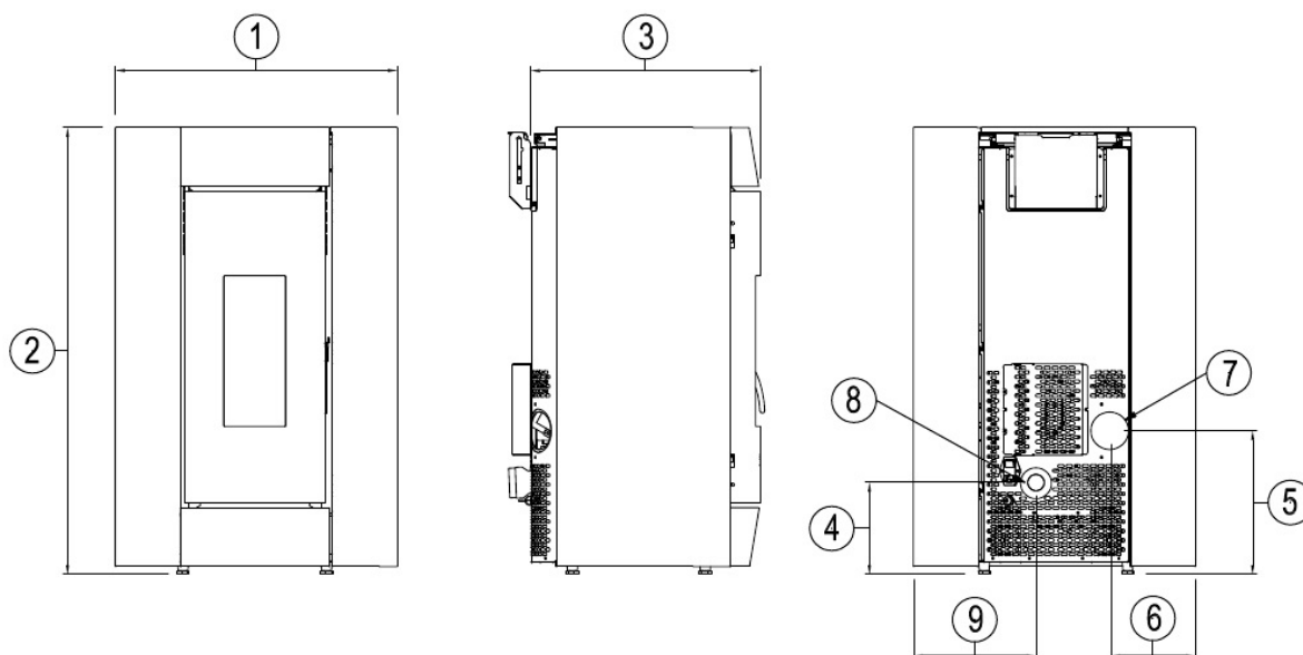
Fig. 20 - Algemene afmetingen: Elise 3
