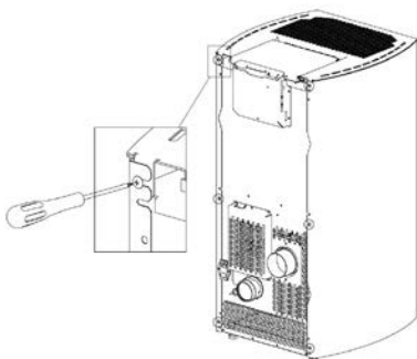
Fig. 56 - Draai de schroeven los
