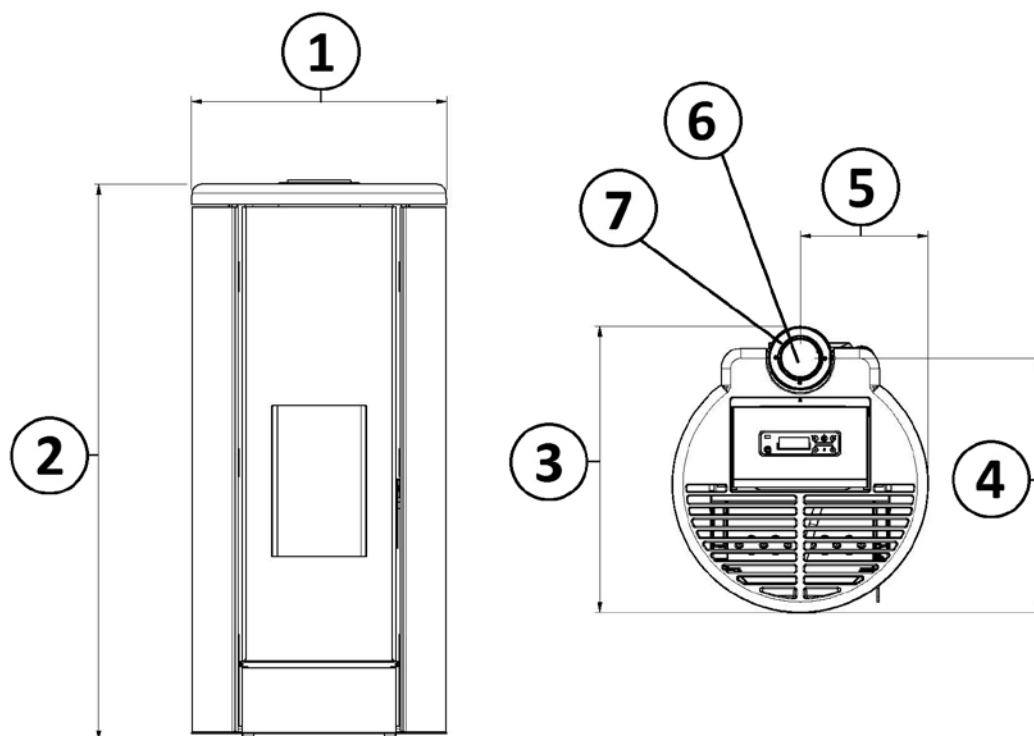
Fig. 29 - Algemene afmetingen: Breeze Airtight
