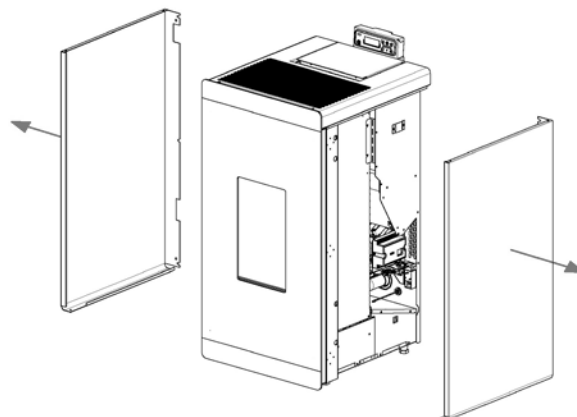
Fig. 71 - Verwijdering zijpanelen
