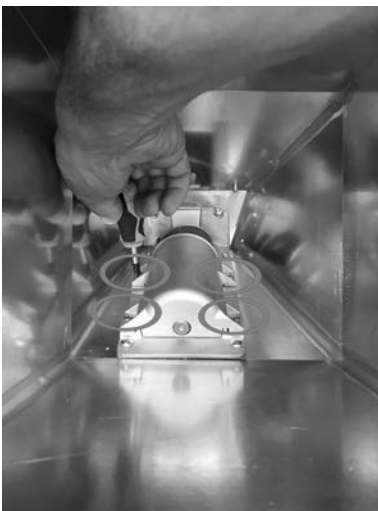
Fig. 80 - Verwijdering van de schroeven
