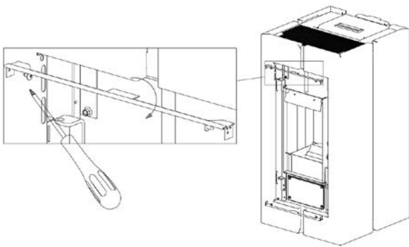
Fig. 54 - Verwijdering profielen
