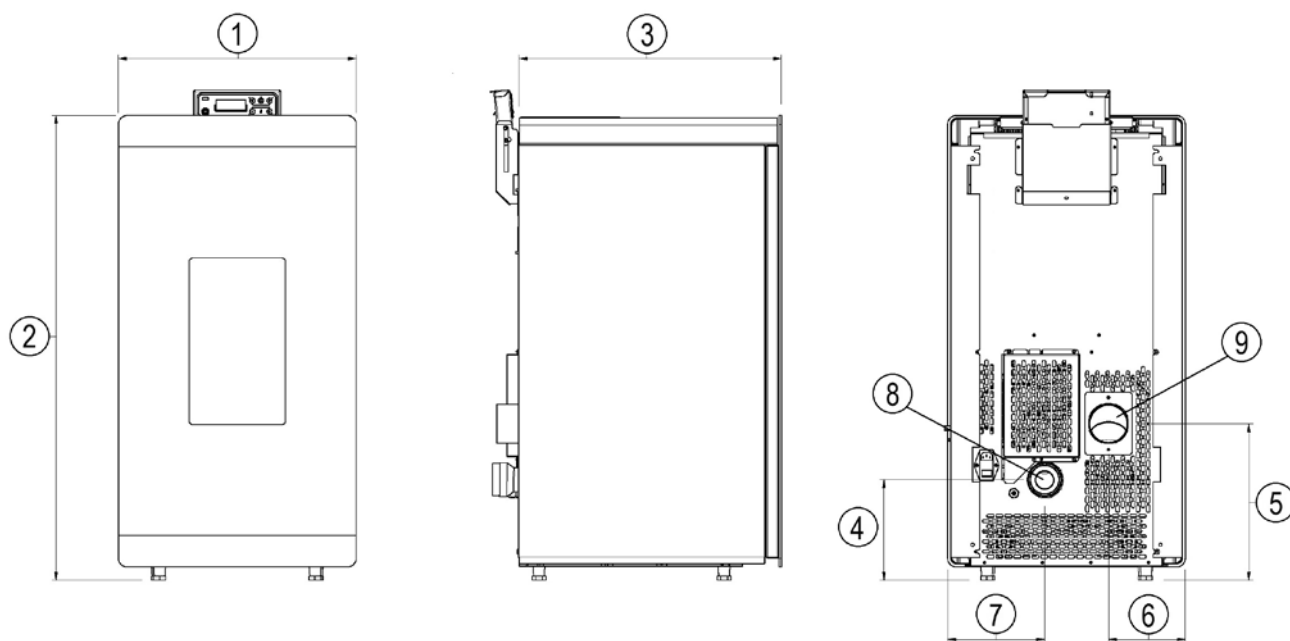
Fig. 22 - Algemene afmetingen: Glass
