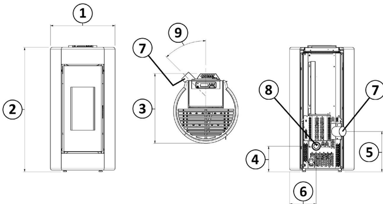
Fig. 21 - Algemene afmetingen: Shell P
