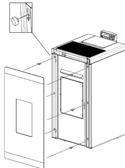
Fig. 42 - Plaats het glas
