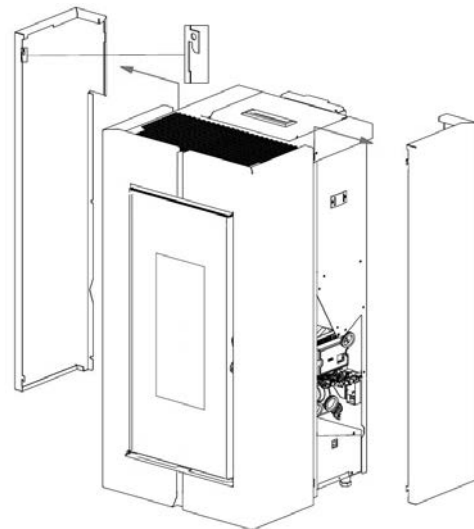
Fig. 53 - De zijpanelen losmaken
