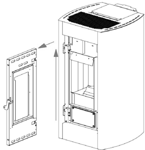
Fig. 33 - Verwijdering van de deur
