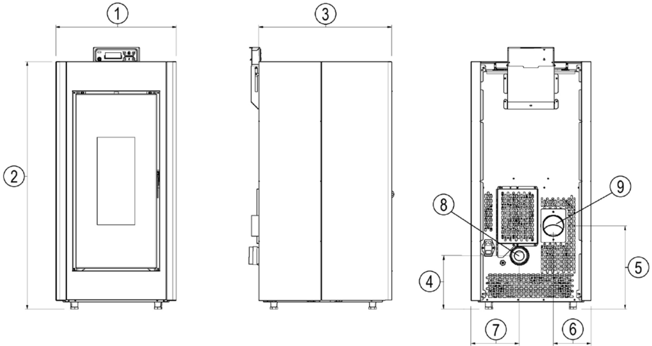
Fig. 23 - Algemene afmetingen: Verve Airtight
